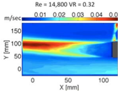
Figure 14. V_{\text{prime}} RMS of med Re.
