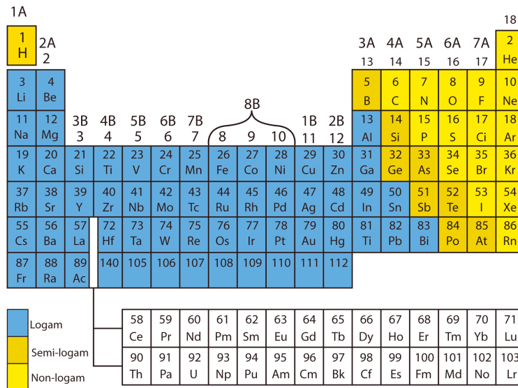
Gambar 3.1 Sistem Periodik Unsur
