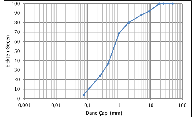
Şekil 16: Zemin numunelerine ait elek analizi grafiği.
