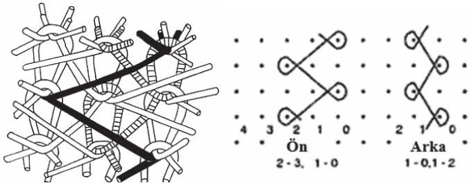
Şekil 2. Çözgümlü kilit örme kumaş yapısı
