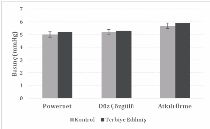
Şekil 4. Kitosan ile terbiye işlemi görmüş numunelerin ortalama final basınçları (mmHg) (hata çubukları: \pm standart sapma)
