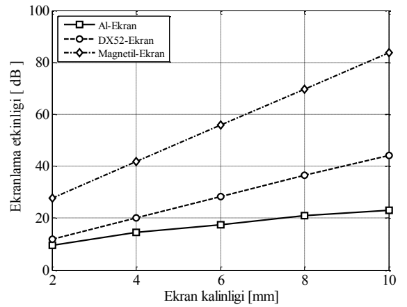
Şekil 7: Ekranlama etkinliğinin ekran kalınlığına bağlı değişimi.
