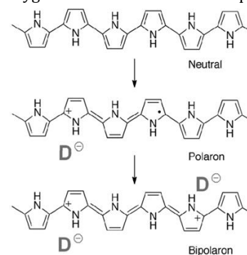
Şekil 2: İletken polimerlerin redoks yapıları.
