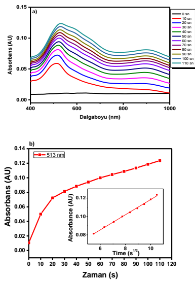
Şekil 11: (a): P(HKCN)'e ait in-situ elektrokimyasal polimerizasyonu, (b): 513 nm dalga boyunda gözlenen zaman-Absorbsans grafiğı. İç grafiğ: 513 nm dalga boyunda zamanın karekökü ile absorbsans değışikliğı grafiğı.
