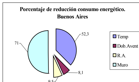
Figura 8: Comparación de la reducción del consumo energético según medidas de mejora de la envolvente. Provincia de Buenos Aires.
