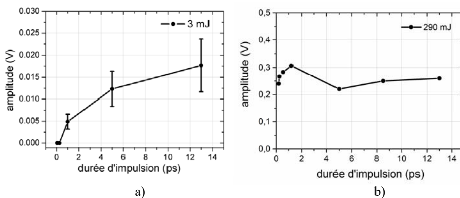
Figure 7. Amplitude signal acoustique en fonction de la durée d'impulsion laser a) faible énergie, b) énergie élevée
