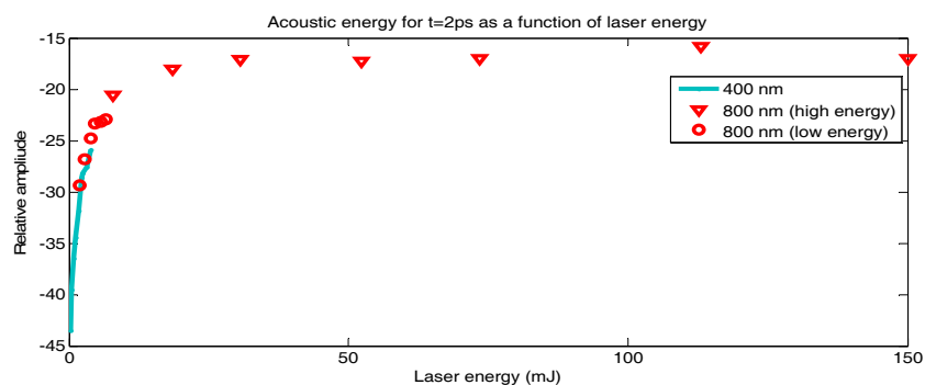
Figure 10. Amplitude du signal acoustique (dB) en fonction de l'énergie laser pour deux longueurs d'ondes différentes (400 nm et 800 nm). La durée d'impulsion est de 2 ps.
