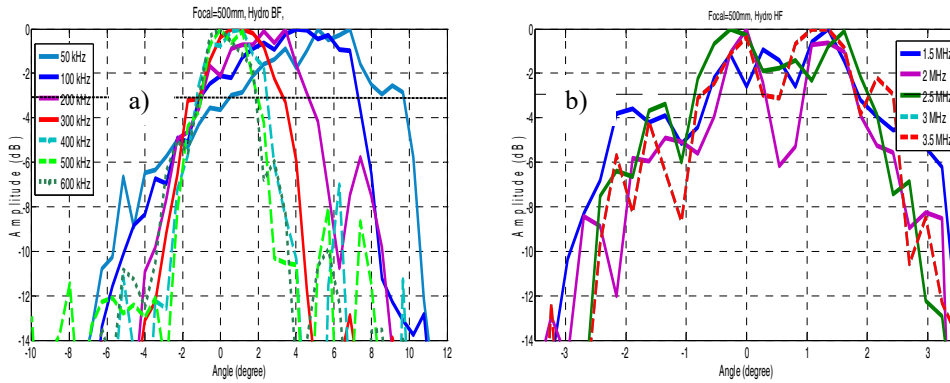
Figure 5. Directivité de la source dans un plan vertical ( f = 500 mm), a) hydrophone Reson TC4035, b) hydrophone Acoustic Precision
