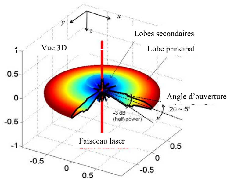
Figure 6. Diagramme 3D de la source acoustique pour la fréquence f = 2 MHz (paramètres laser : E = 290 mJ, durée d'impulsion \tau = 1 ps, focale = 200 mm)
