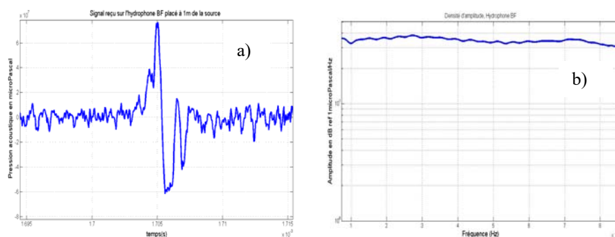
Figure 3. a) Signal acoustique reçu par l'hydrophone Reson TC4035 et b) niveau acoustique calculé par FFT du signal reçu. (Correction par la réponse fréquentielle du transducteur)
