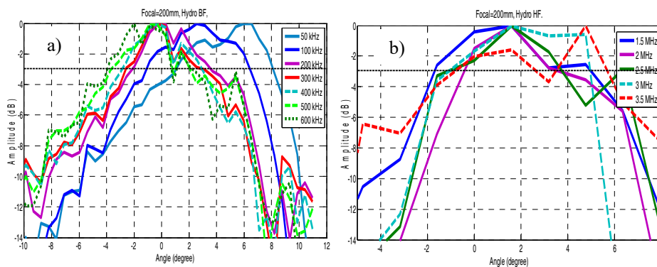
Figure 4. Directivité de la source dans un plan vertical ( f = 200 \text{ mm} ), a) hydrophone Reson TC4035, b) hydrophone Acoustic Precision
