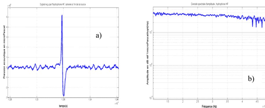
Figure 2. a) Signal acoustique reçu par l'hydrophone AP, ramené à 1 m de la source, et b) niveau acoustique calculé par FFT du signal reçu. (Correction par la réponse fréquentielle du transducteur)
