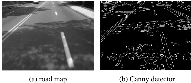
Figure 2. Edge detection
