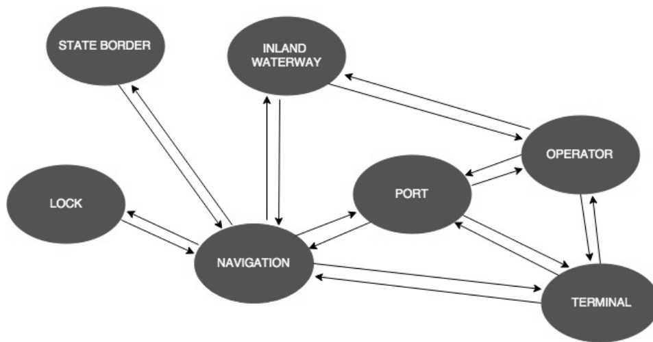
Fig. 3. Arrangement and communication of Agents in the system Rys. 3. Rozmieszczenie i komunikacja agent w systemie
