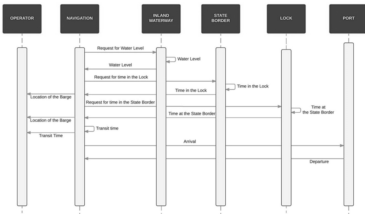
Fig. 4. Agents' communication at Navigation Rys. 4. Komunikacja agent w nawigacji
