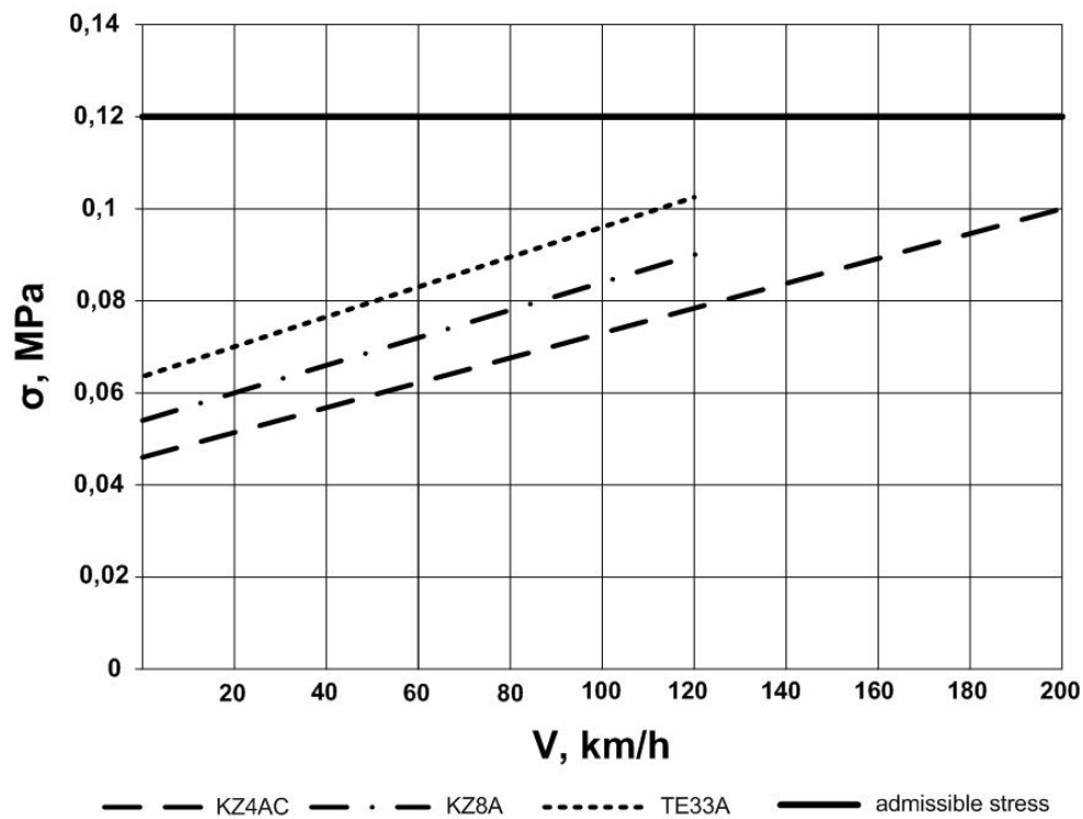
Fig. 5. Stress in the road bed Рис. 5. Напряжение в земляном полотне
