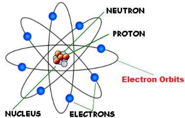
Modelo atómico de Rutherford (1910's)
