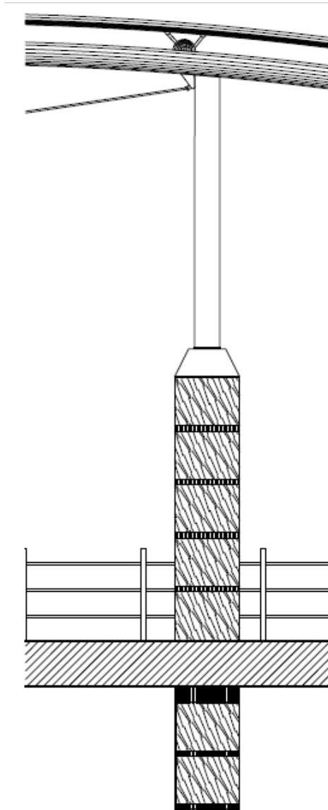
Imagen 36: Detalle constructivo columna que soporta cubierta
