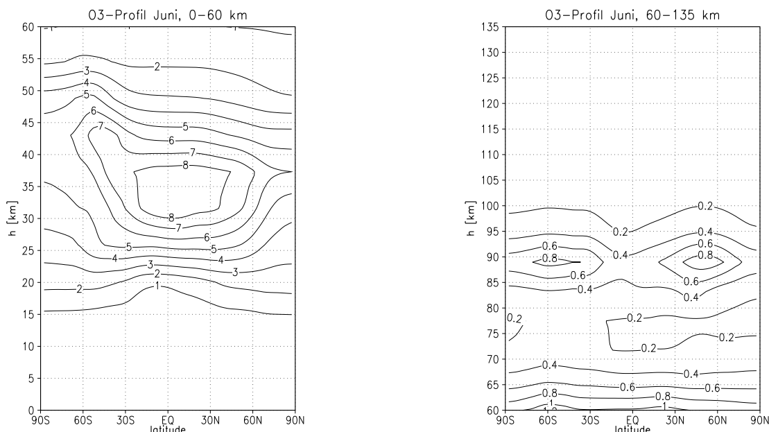
Abbildung 2.1: Ozonprofil in ppmV im COMMA-Modell für Juni abgeleitet aus einer erweiterten Version der Berliner Ozonklimatologie nach Fortuin und Langematz (1994).
