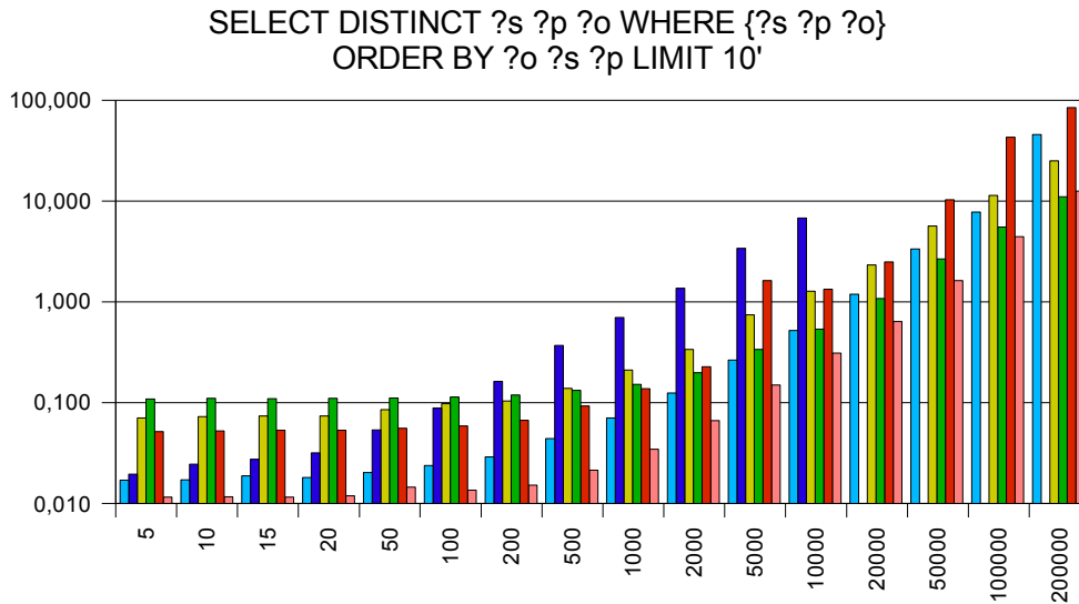
Abbildung 6.6: Sortieren auf distinkten Tripeldaten
