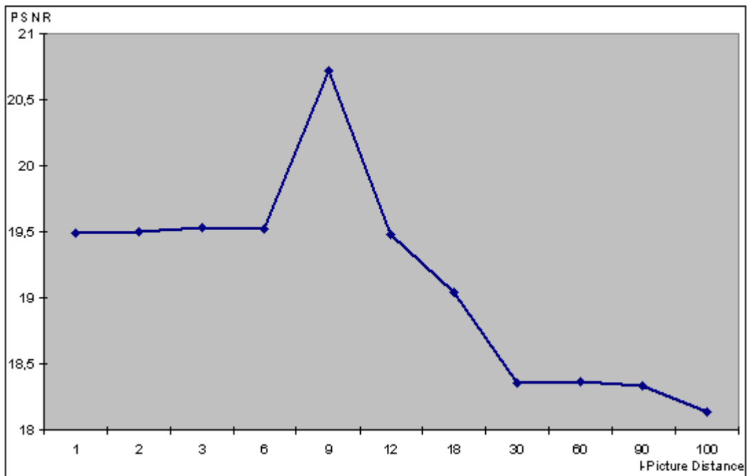
Abbildung 6-23 PSNR- Werte für MPEG 2, 3000 kbit/s, (I = 3-100, P = 1)
