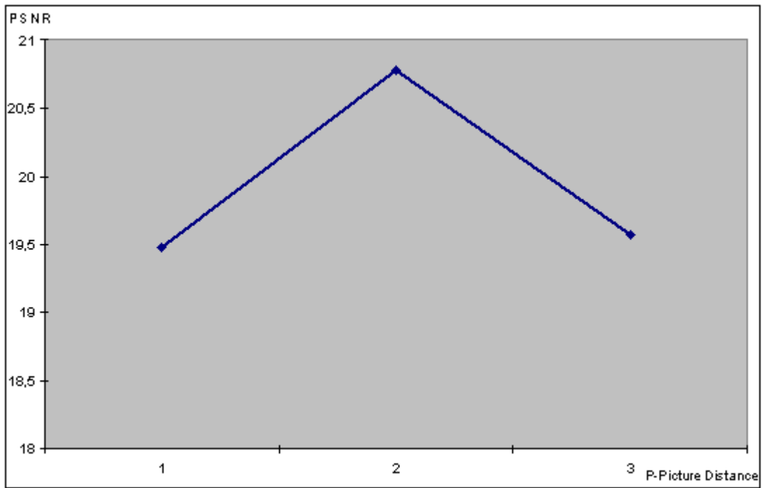
Abbildung 6-24 PSNR- Werte für MPEG 2, 3000 kbit/s, (I = 12, P = 1-3)
