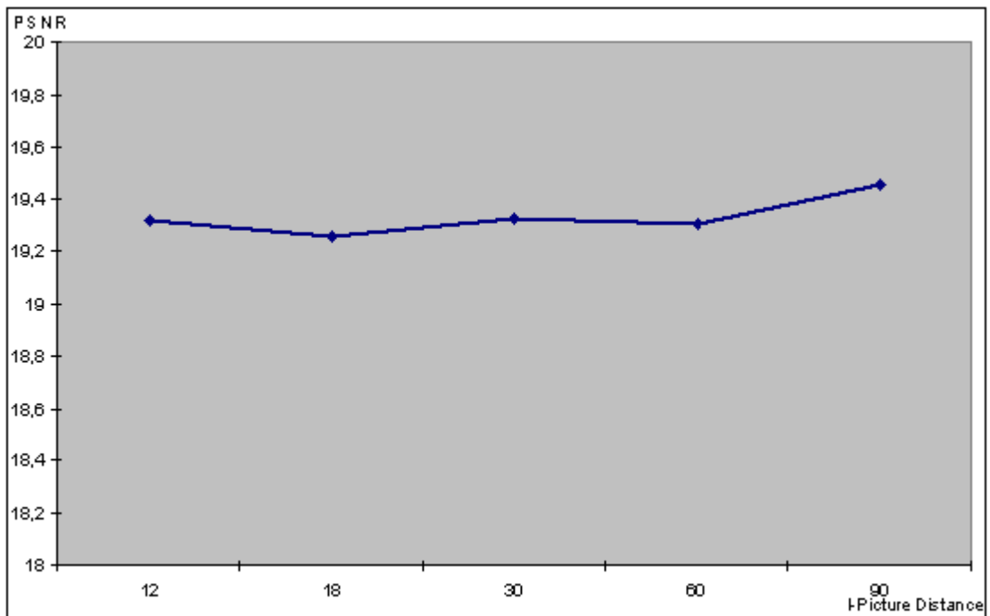
Abbildung 6-11 PSNR- Werte für MPEG 1, 760,4 kbit/s, (I = 12-90, P = 1)
