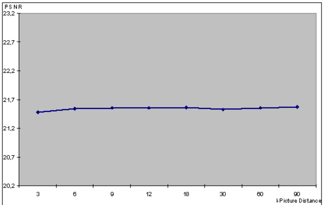
Abbildung 6-21 PSNR- Werte für MPEG 2, 2000 kbit/s, (I = 3-90, P = 3)
