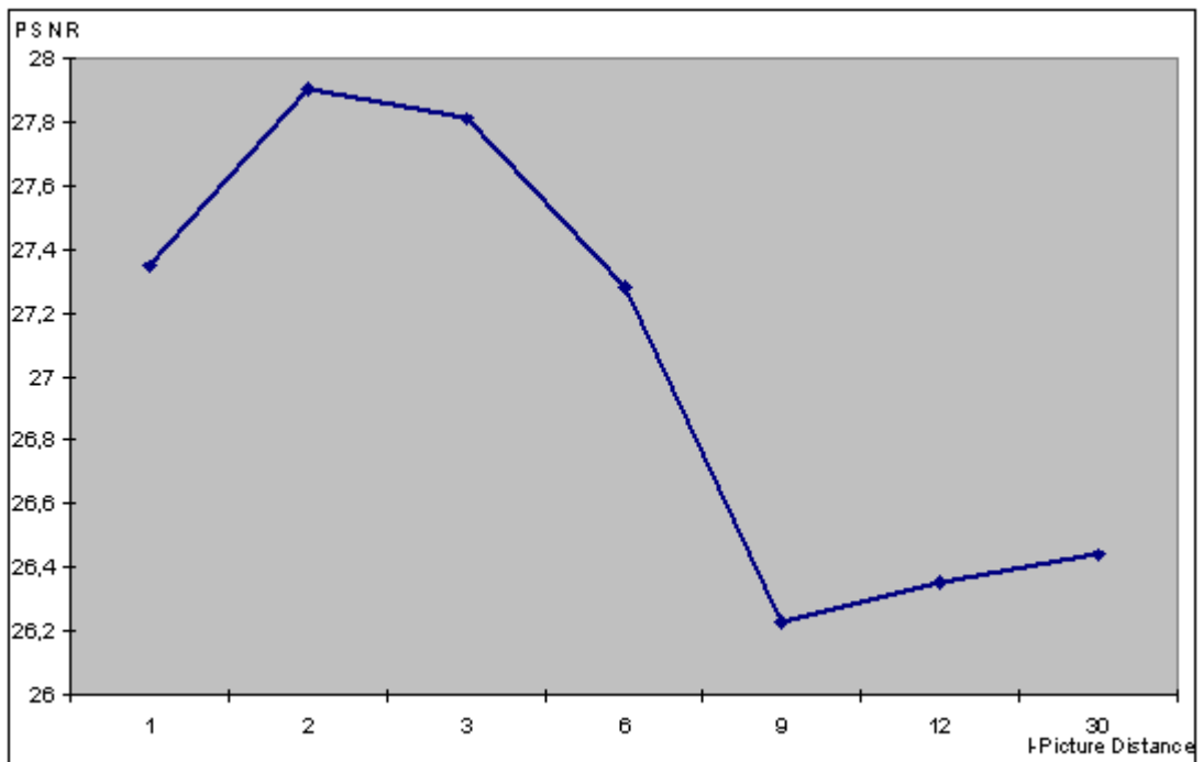
Abbildung 6-17 PSNR- Werte für MPEG 1, 3000 kbit/s, (I = 1-30, P = 1)
