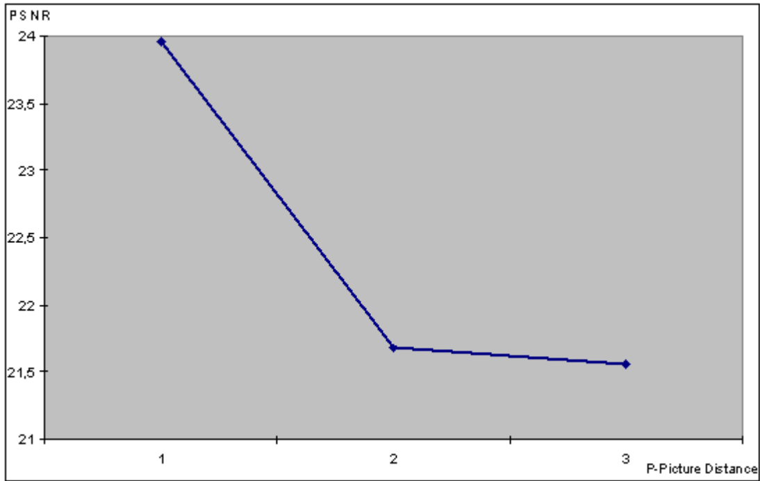
Abbildung 6-20 PSNR- Werte für MPEG 2, 2000 kbit/s, (I = 12, P = 1-3)
