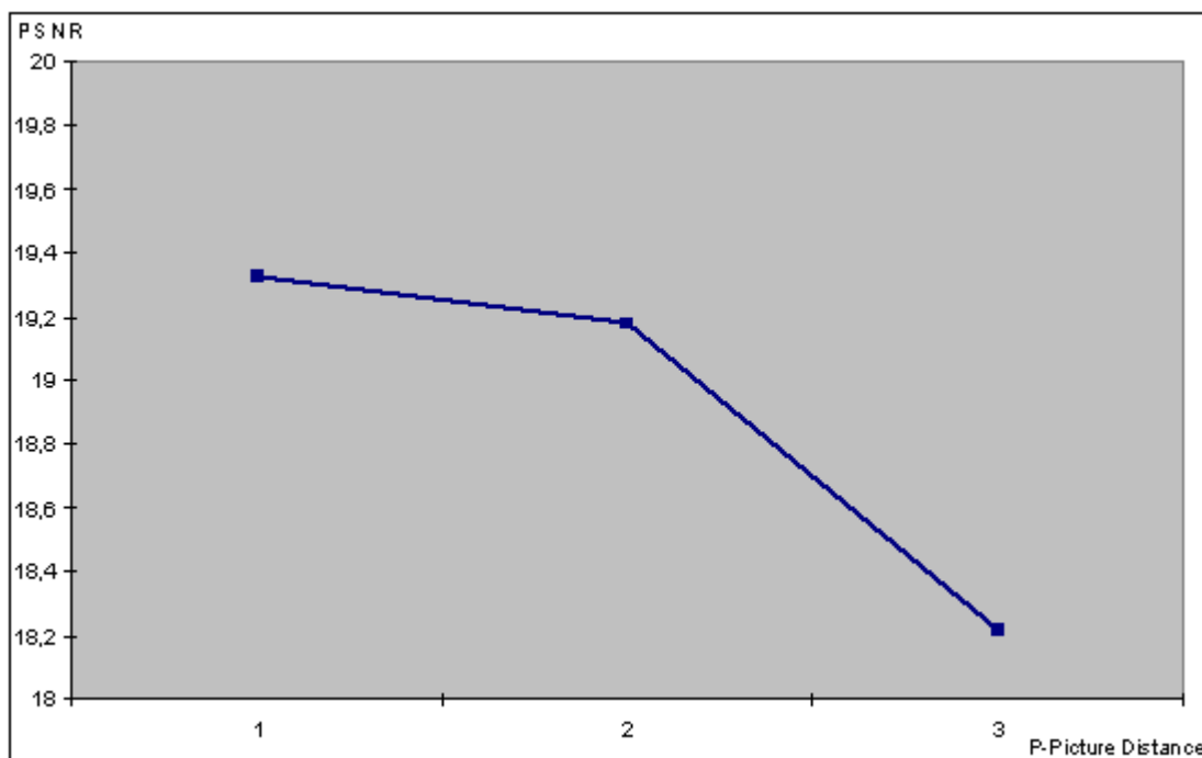
Abbildung 6-9 PSNR- Werte für MPEG 1, 760,4 kbit/s, (I = 12, P = 1-3)
