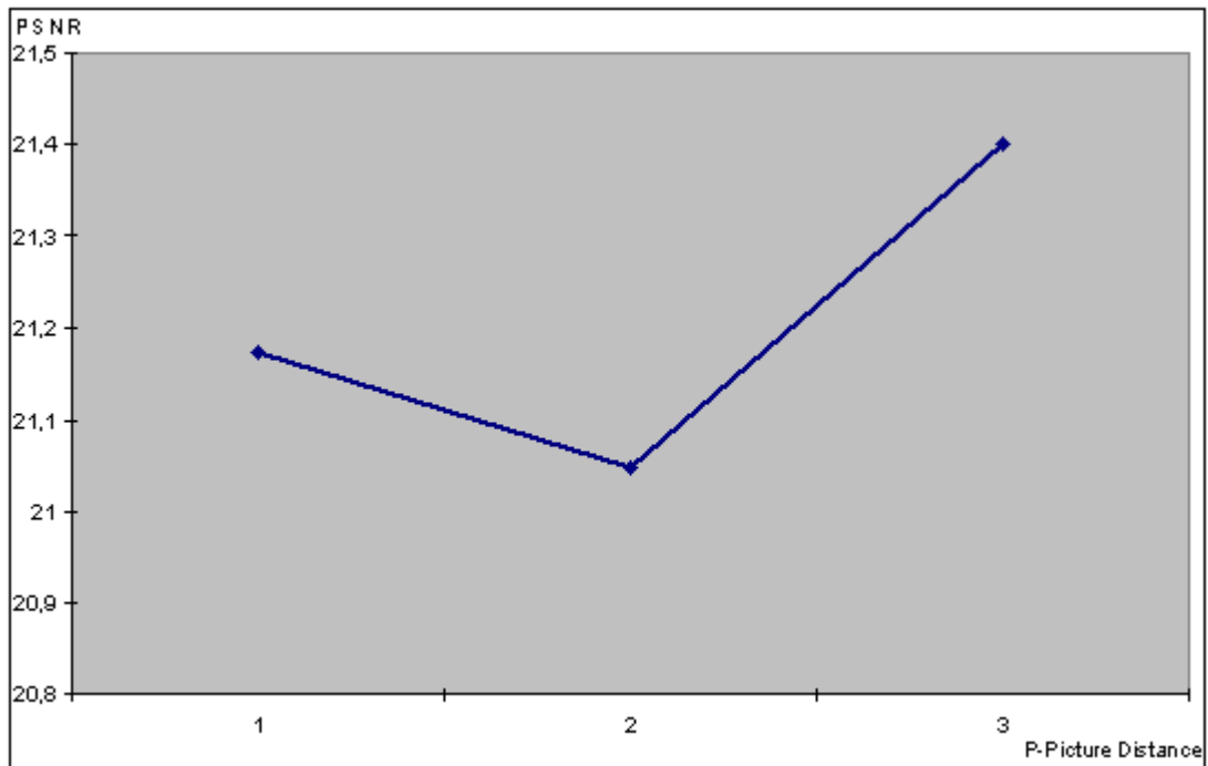
Abbildung 6-14 PSNR- Werte für MPEG 1, 2000 kbit/s, (I = 12, P = 1-3)
