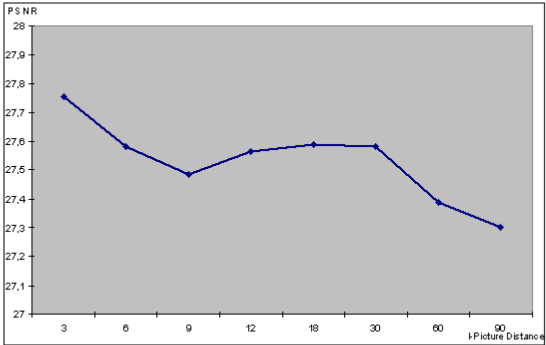
Abbildung 6-16 PSNR- Werte für MPEG 1, 3000 kbit/s, (I = 3-90, P = 3)
