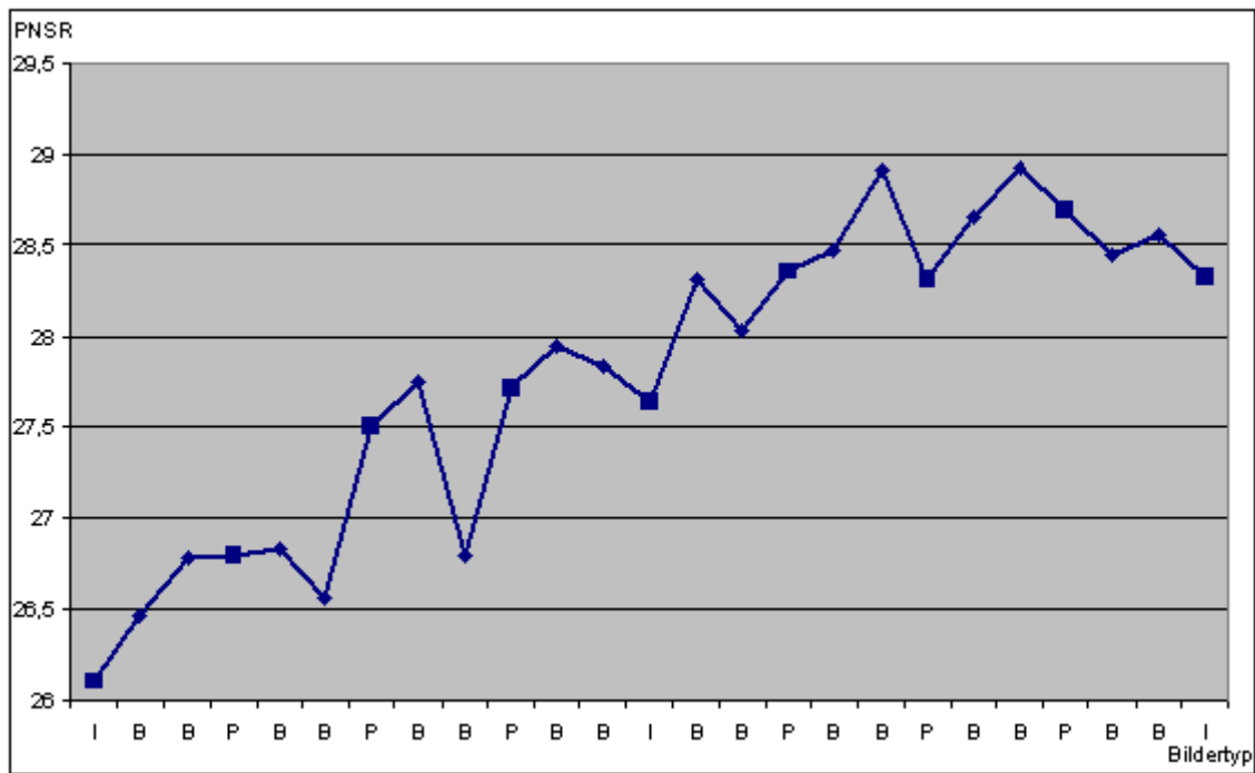
Abbildung 6-8 PSNR Entwicklung I=12 P=3 (MPEG1 760,4kbit/s)
