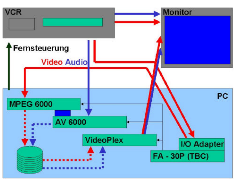
Abbildung 5-3 Die Komponenten im Zusammenspiel
