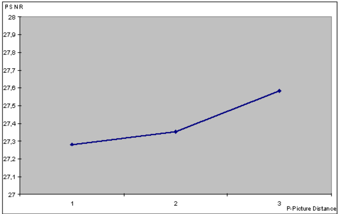
Abbildung 6-18 PSNR- Werte für MPEG 1, 3000 kbit/s, (I = 6, P = 1-3)
