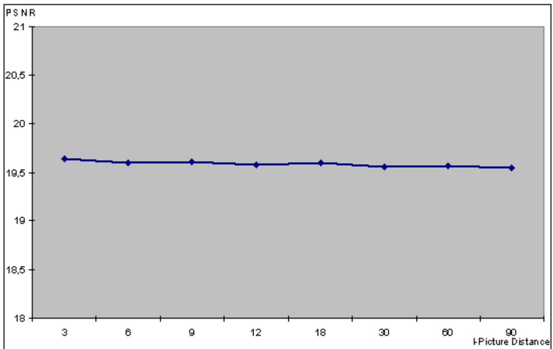
Abbildung 6-25 PSNR- Werte für MPEG 2, 3000 kbit/s, (I = 3-90, P = 3)
