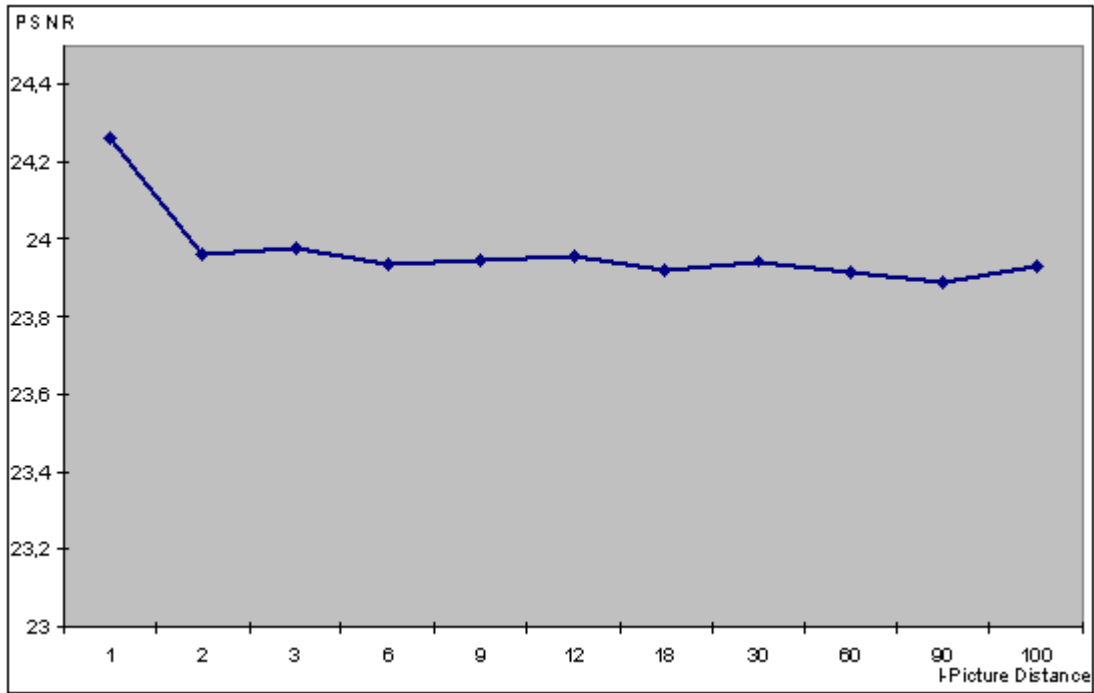
Abbildung 6-22 PSNR- Werte für MPEG 2, 2000 kbit/s, (I = 1-100, P = 1)
