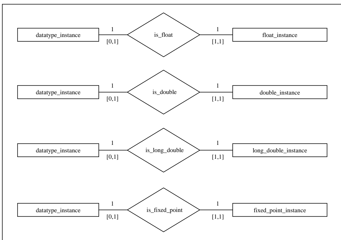
Abbildung A-3: Entities und Relationships zur Darstellung von Werten von numerischen, nicht-ganzzahligen IDL-Typen.
