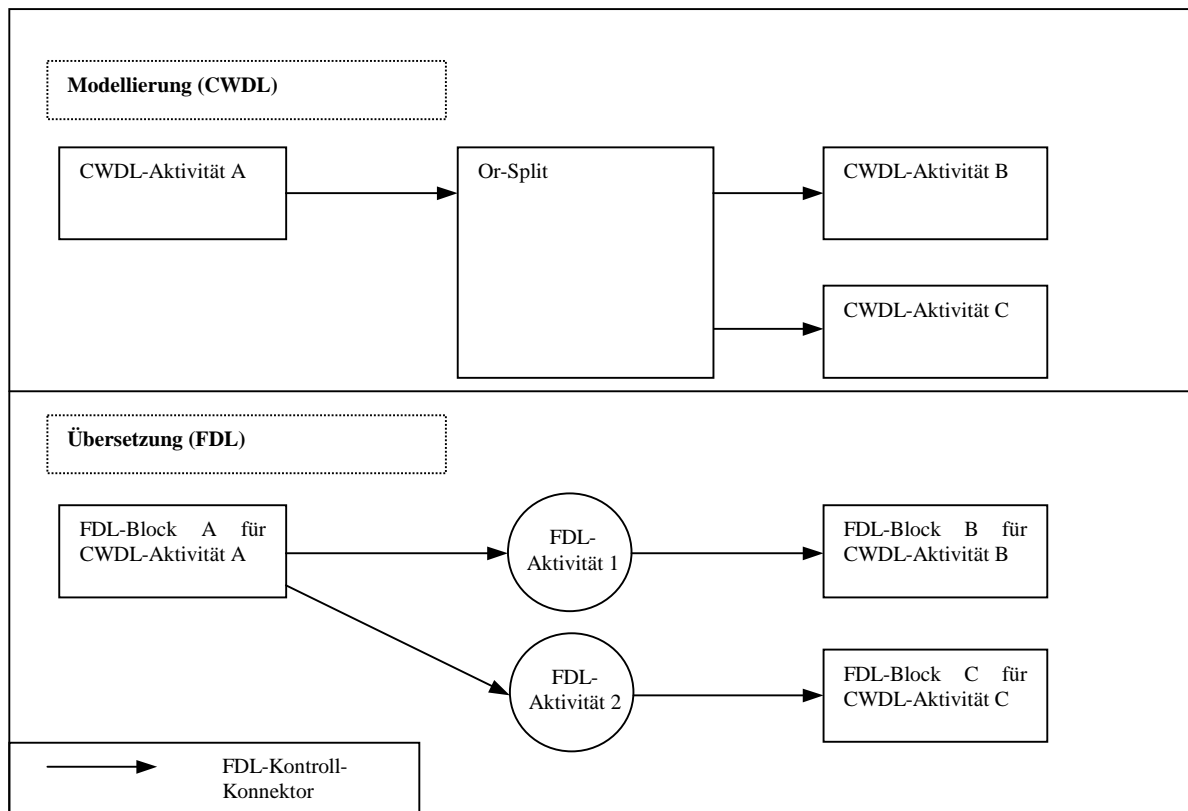
Abbildung 3-12: Die Übersetzung eines CWDL-Or-Splits.
