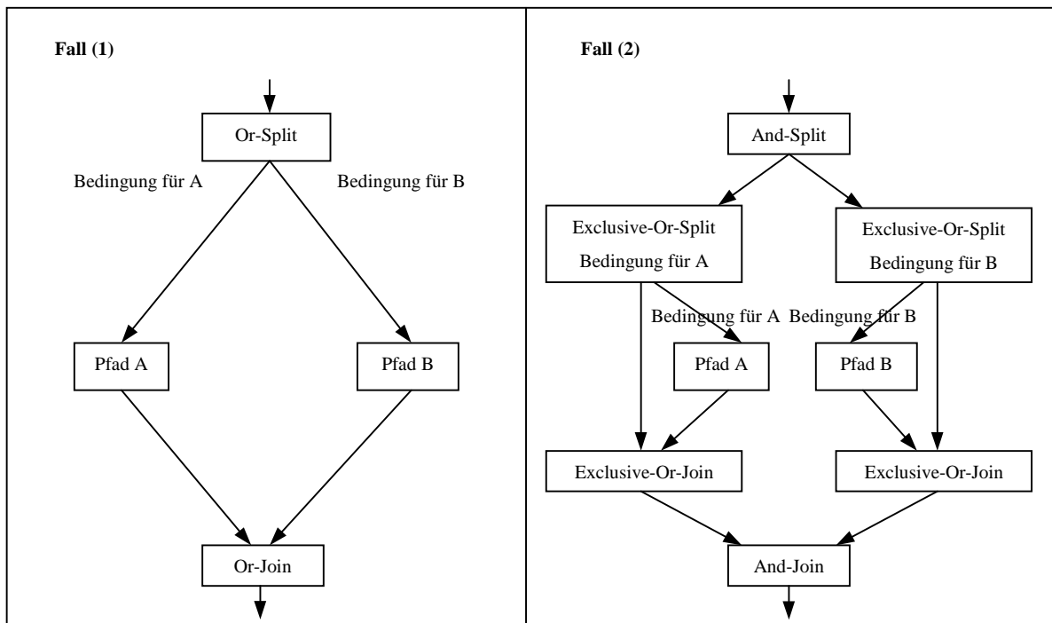
Abbildung 3-3: Logische Operatoren im Kontrollfluß.
