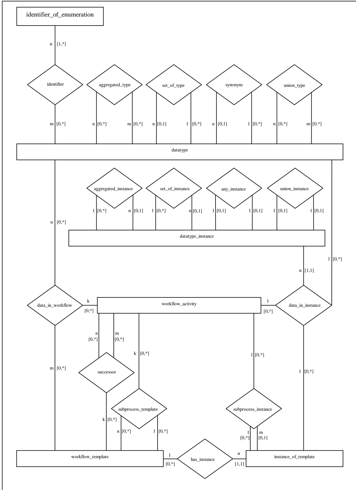
Abbildung A-1: Entity-Relationship-Diagramm für die Darstellung von IDL-Datentypen.
