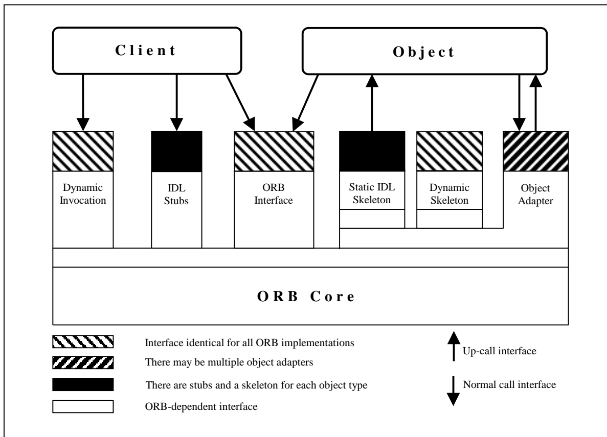
Abbildung 2-1: CORBA: Basiselemente. Nach [OMG98].
