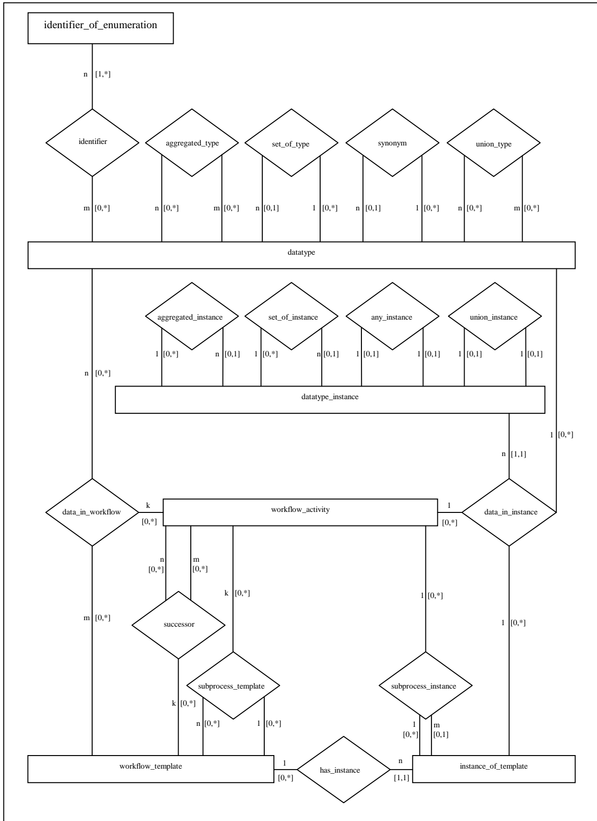
Abbildung 3-4: Die Darstellung von IDL-Datentypen in einer Datenbank.
