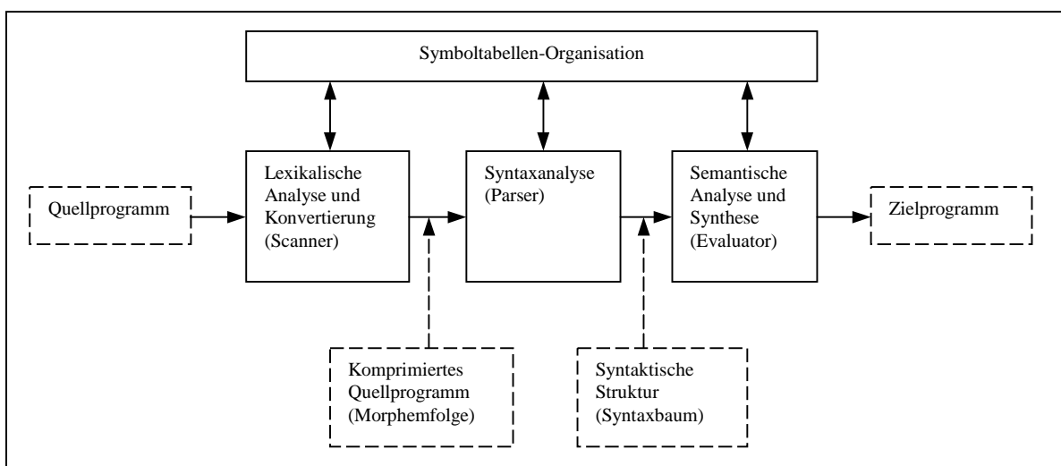
Abbildung 4-2: Logische Struktur eines Compilers. Nach [LJO87].
