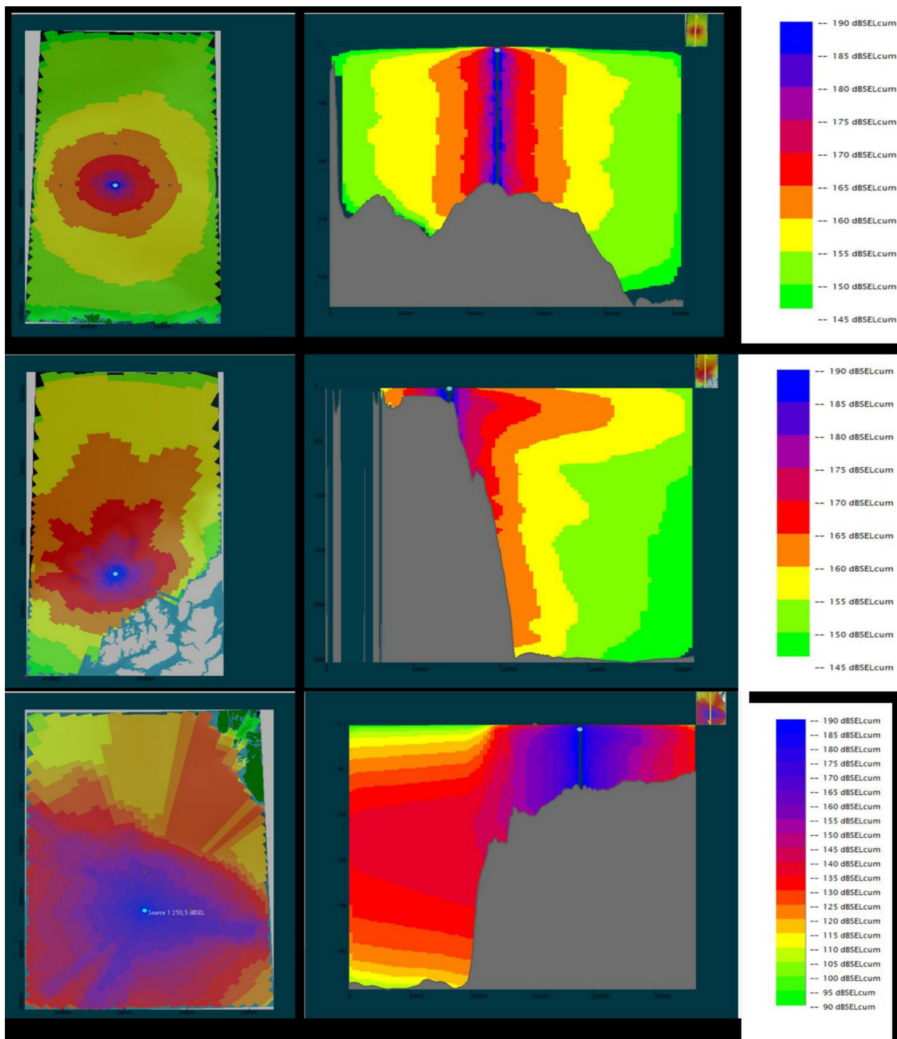
Figur A2.4. Screenshots for Nordkappbanken (øverst), Vesterålen (midten) og Nordsjøen sør (nederst). Alle viser snitt sett ovenfra til venstre og tvversnitt til høyre. Merk at for skalaen for Nordsjøen er annerledes enn for de to andre.
