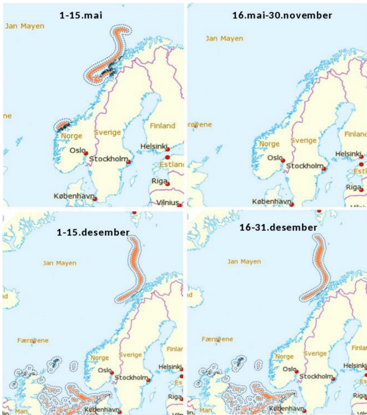
Figur A1.1. Frarådingsoner for seismikkundersøkelser basert på viktige gytefelt og konsentrerte vandringsruter inn mot gytefelt med bufferzoner (5 og 20 nmi) for alle perioder gjennom året. Fra 1.mai – 30.nov foregår det ikke gyting i særlig grad, og det er da ingen områder som frarådes.
