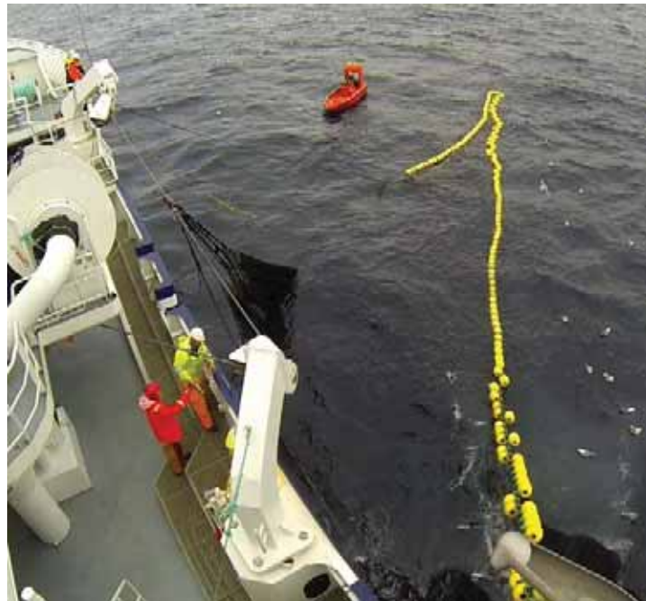
Figur 14. Geila er åpnet for å slippe ut fisk, men blir delvis stengt igjen av en not-fold som strekker seg ut fra den nederste ringen.
