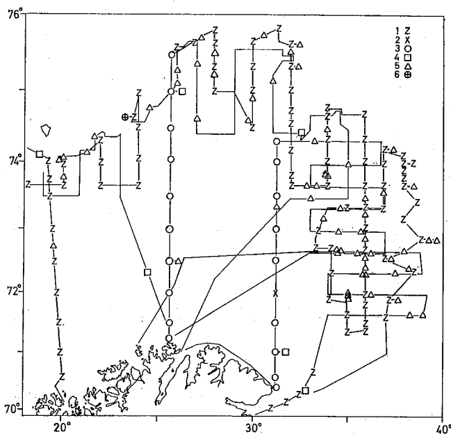
Fig. 1. Kurser og stasjoner 19. nov.—11. des. 1) Hydrografisk st. med TS sonde, 2) hydrografisk st. med bathytermograf, 3) hydrografisk st. med vannhenter, 4) bunntårlst., 5) pelagisk trålst., 6) snurp. [Survey route and grid of station 19 Nov.—11 Dec. 1) Hydrographic st. with TSD sonde, 2) hydrographic st. with bathythermograph, 3) hydrographic st. with water bottles, 4) bottom trawl st., 5) pelagic trawl st., 6) purse seine st.].
