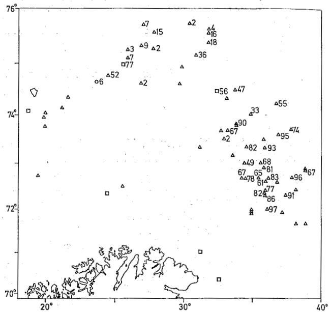
Fig. 4. Vektprosent modnende lodde i trållfangstene. [Maturing capelin in weight percent in the trawl catches].
