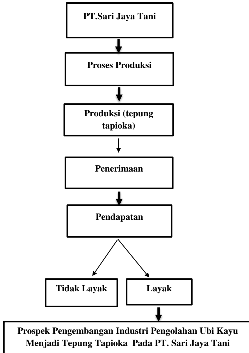
Gambar 1 Kerangka Pemikiran
