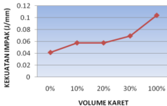
Gambar 3. Hubungan kekuatan impak terhadap volume karet
