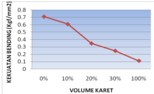
Gambar 2. Hubungan kekuatan bending terhadap volume karet
