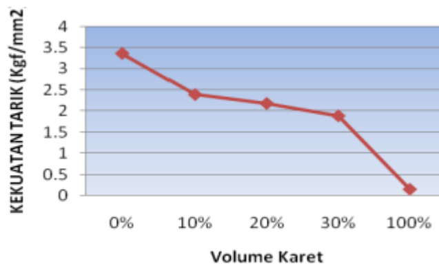
Gambar 1. Hubungan kekuatan tarik terhadap volume karet
