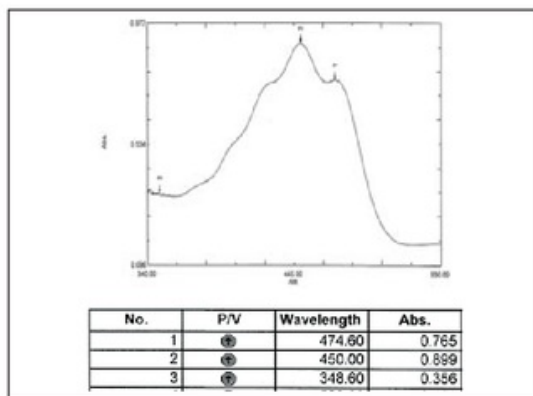
Gambar 3. Spektra \beta -karoten standar pada spektrofotometri UV-Vis
