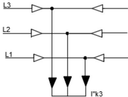
Figura 4 Cortocircuito trifásico (Inlernationale & Commission, 2001). Adaptado por D. Novoa, 2019.
