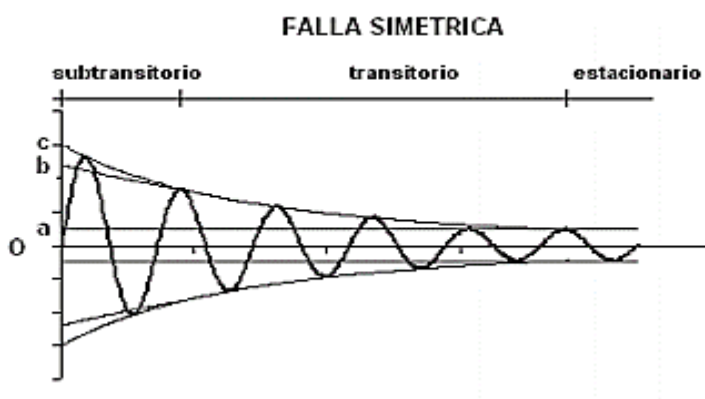
Figura 10 Composición de una corriente de cortocircuito simétrica (Farfán, 2003)
