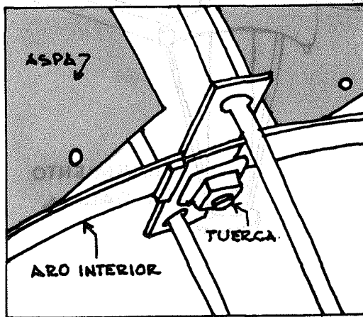
DETALLE 2 UNION DE LOS BRAZOS CON EL ARO INTERIOR
