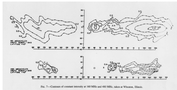
(b) Mapas de contorno presentados por Reber (Reber 1949). Las áreas más brillantes corresponden a la Vía Láctea.
