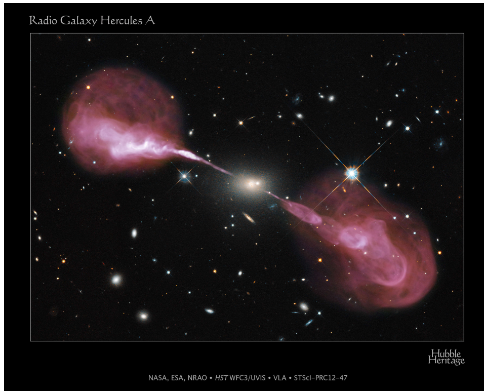
Figura 1.9: Imagen de luz visible obtenida por el Telescopio Espacial Hubble superpuesta con una imagen de radio tomada con el radio interferómetro JVLAs.
