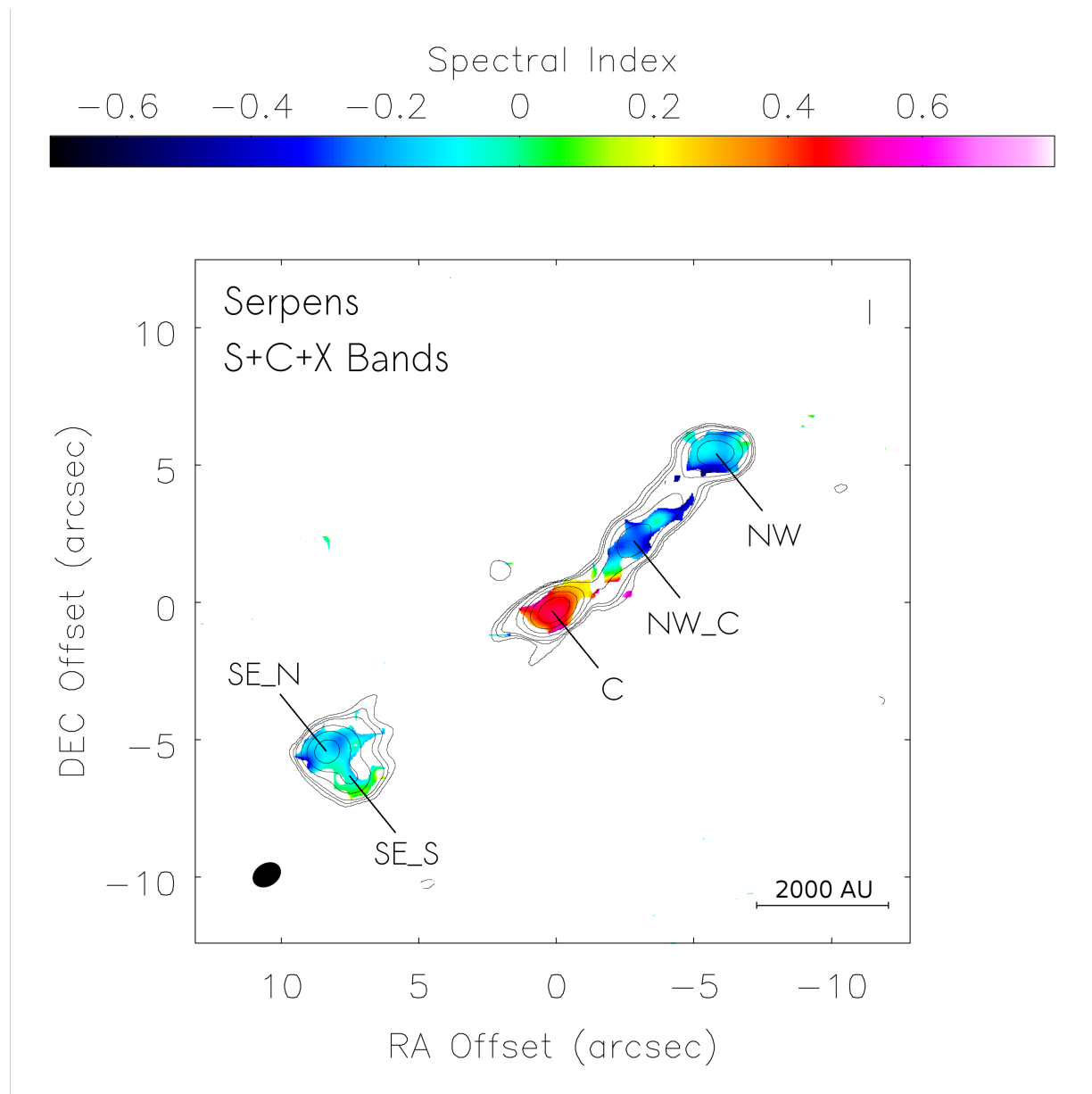
Figura 3.1: Superposición de la imagen en radio continuo realizada con datos combinados de bandas S, C, y X correspondientes a la época 2012 (contornos) sobre la imagen de índice espectral (escala de color). Los contornos corresponden a -4 , 4 , 6 , 8 , 16 , 31 , 64 , y 128 veces el rms de la imagen en radio continuo, 6\mu\text{Jy}/\text{beam} . El haz sintetizado es 1.07'' \times 0.80'' con un PA de -58^\circ . Los píxeles que se muestran en la imagen de índice espectral son aquellos para los cuales el error en el índice espectral es menor que 0.1 . Las fuentes discutidas en este trabajo (fuente central C, y los nudos externos, SE_N, SE_S, NW y NW_C) se indican en la Figura.
