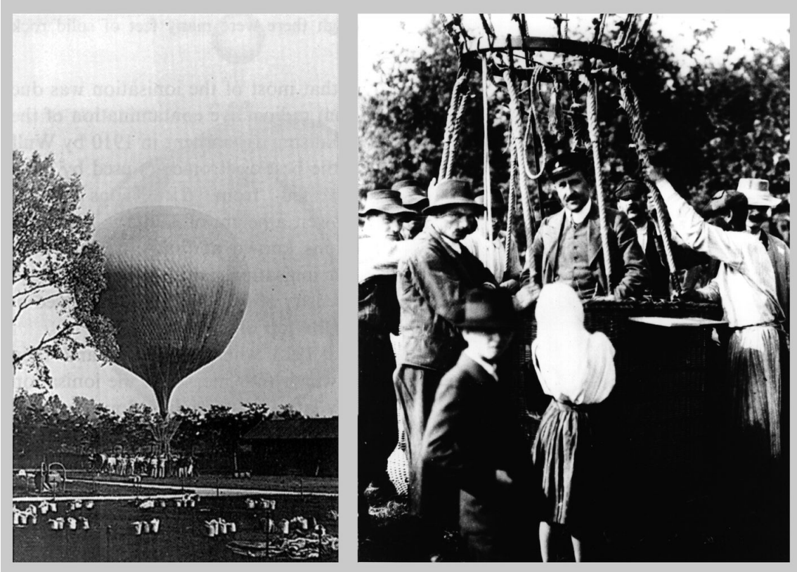
Figura 1.13: Vuelos en globo aerostático de Victor F. Hess. Izquierda: Preparación para uno de sus vuelos en el período 1911-1912. Derecha: Hess después de unos de sus exitosos vuelos en los cuales se descubrió el incremento de la ionización atmosférica con la altura. (De Y. Sekido y H. Elliot eds 1985. Early history of cosmic rays studies , Dordrecht: D. Reidel Publishing Company.)
