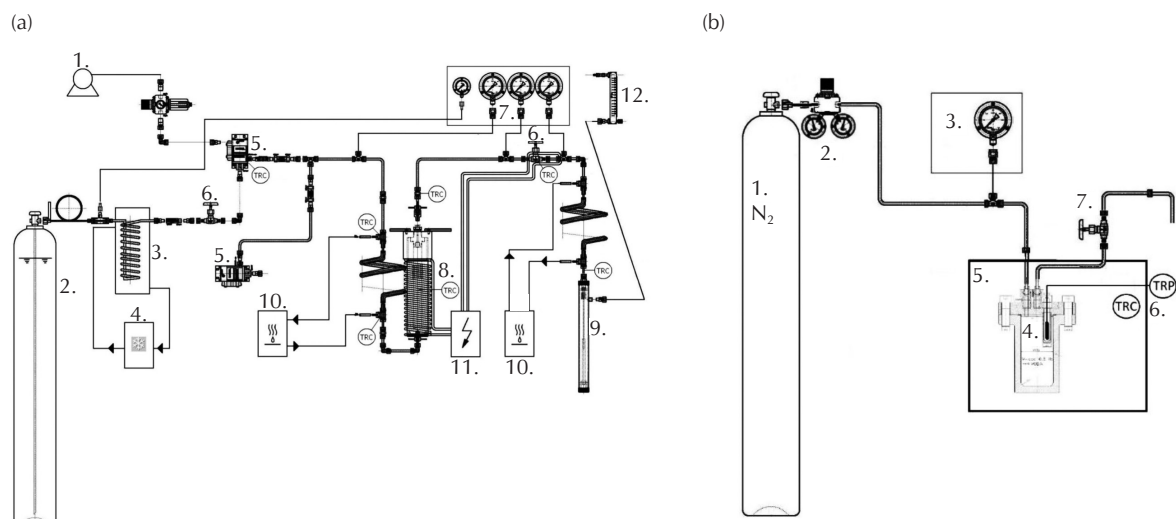
Slika 2 – Procesna shema uređaja: (a) za ekstrakciju superkritičnim CO 2 (1. Kompresor; 2. CO 2 spremnik; 3. Izmjenjivač toplote od nehrđajućeg čelika; 4. Rashladna kupelj; 5. Zrakom pogonjena hidraulična pumpa Haskel MS-71; 6. Ventili (B-HV); 7. Manometri; 8. Ekstraktor; 9. Separator; 10. Vodena kupelj; 11. Centralizirani sistem grijača od staklenih vlakana; 12. Mjerač protok) te (b) za ekstrakciju s vodom u supkritičnom stanju (1. boca N 2 ; 2. Regulator N 2 20/5 Mpa; 3. Manometar 0-20 Mpa; 4. Ekstraktor 20 MPa, 200 °C; 5. Termostat ili pećnica 20 – 300 °C; 6. TRC – Temperature regulator controller; TRP – Temperature regulated probe; regulator temperature i temperaturna sonda; 7. Visokotlačni igličasti ventil).
