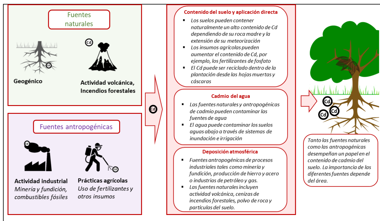
Figura 3 Posibles fuentes de entrada de cadmio a los suelos de cultivo de cacao
