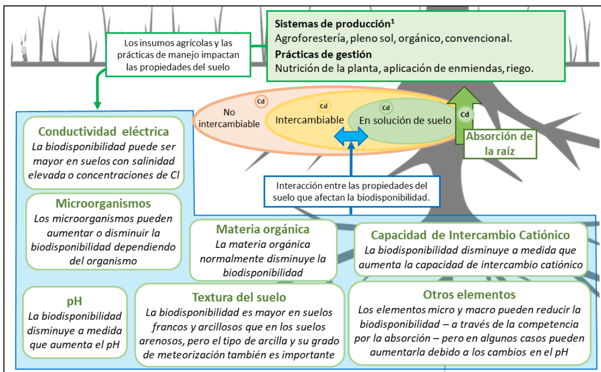
Figura 5 Propiedades del suelo que afectan la disponibilidad de cadmio para las plantas de cacao
