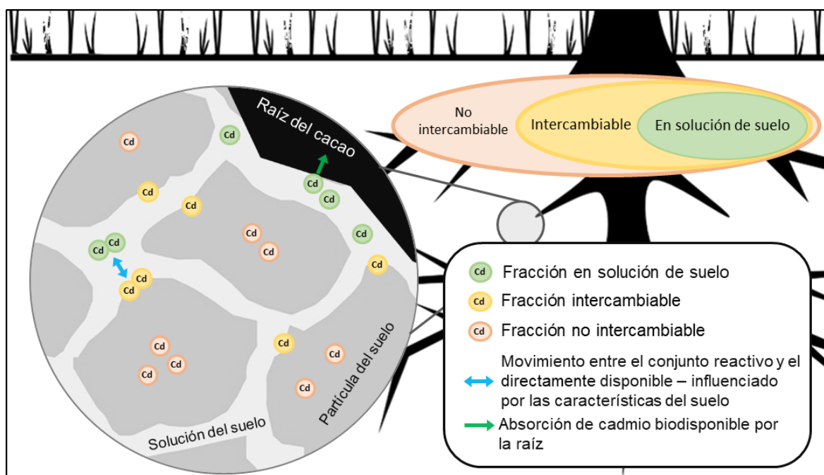
Figura 4 Fracciones de cadmio y biodisponibilidad en suelos [03]
