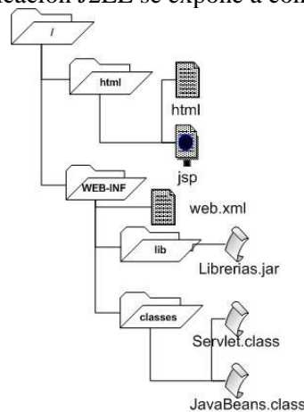
1.Figura 1. Estructura de proyecto web.
