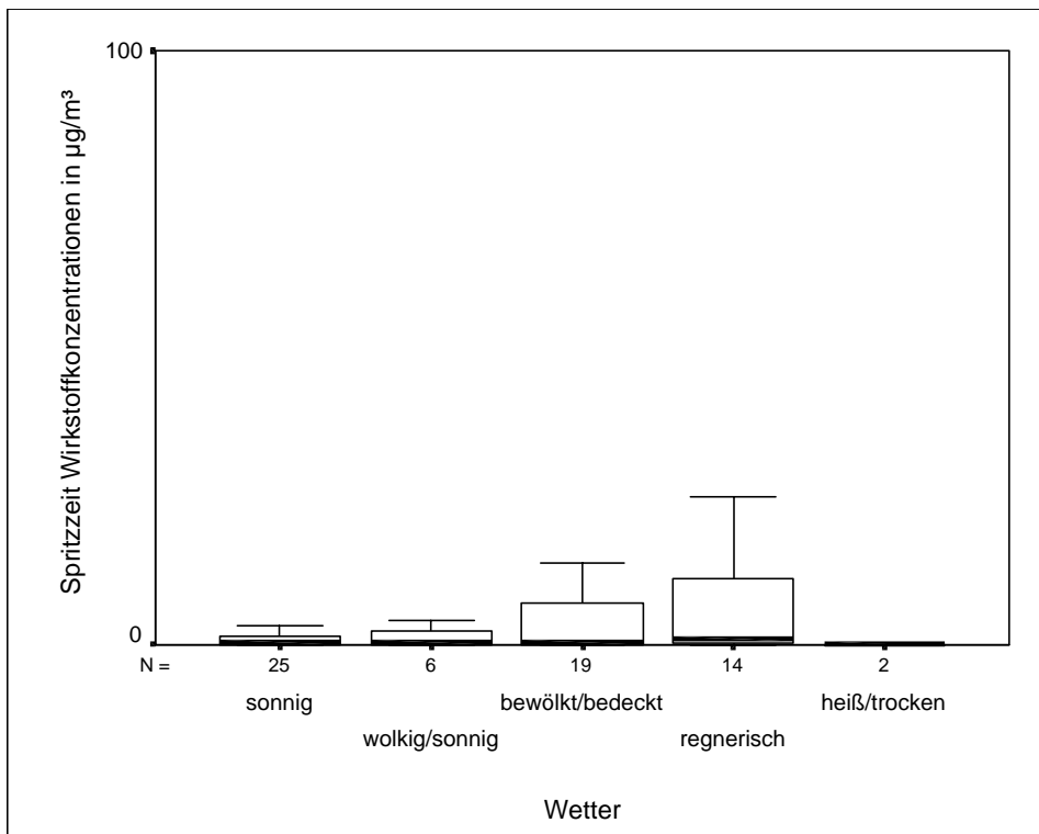
Abb. 4.10 Wettereinfluss auf die inhalative Belastung ( \mu\text{g}/\text{m}^3 ) im Obstbau
