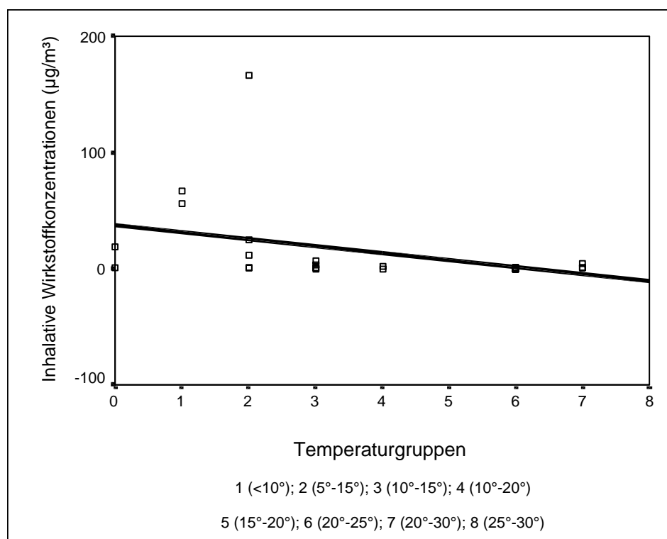
Abb. 4.8 Korrelation zwischen der Temperatur (°C) und der inhalativen Gesamtbelastung (µg/m 3 ) im Obstbau bei Dithiocarbamatexposition
