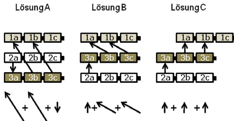
Abb. 5: Drei alternative Lösungen für die Gleiszuordnung
