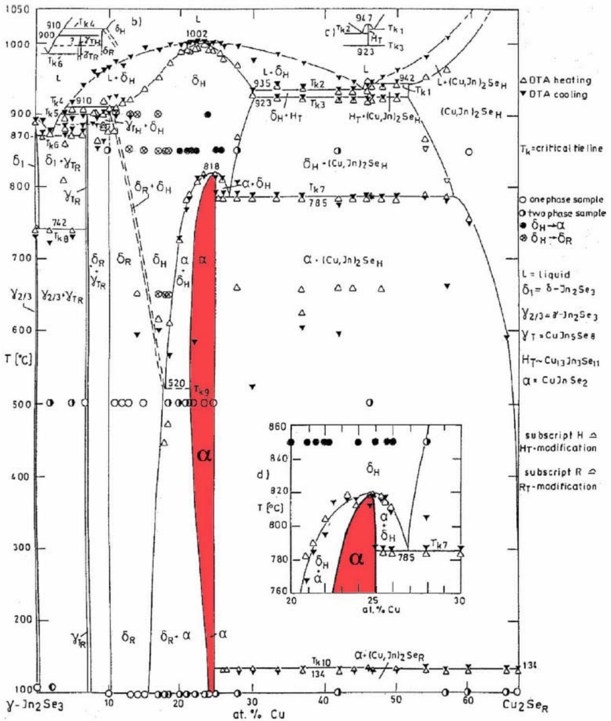
Abb. A.4.: Pseudobinäres Phasendiagramm zwischen \text{Cu}_2\text{Se} und \text{In}_2\text{Se}_3 . Übernommen aus [CLE + 05].
