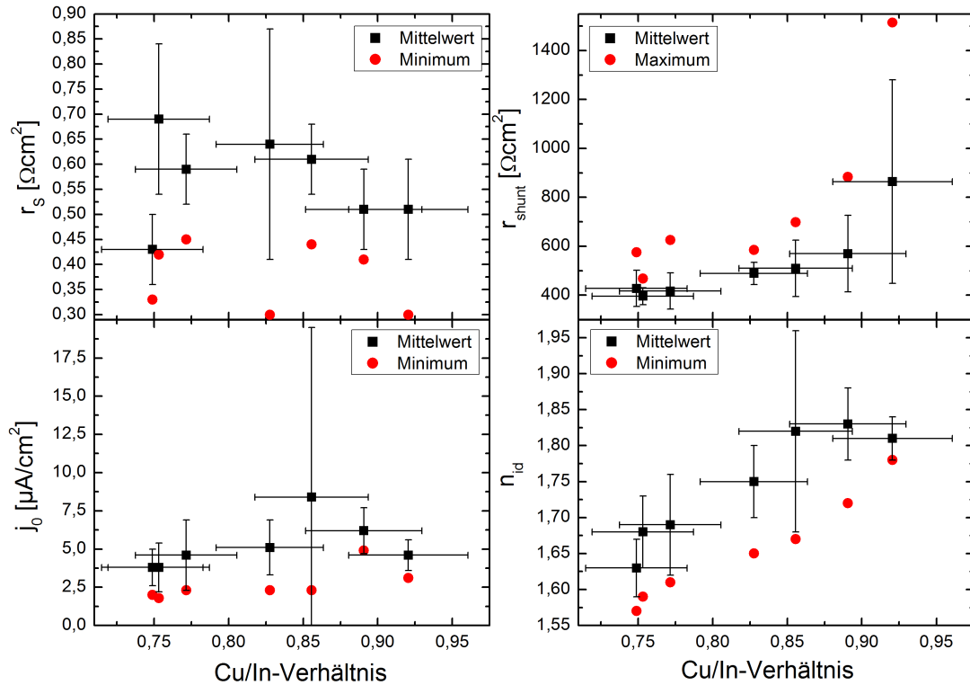
Abb. 7.2.: Graphische Darstellung des spez. Serienwiderstandes r_s (l.o.), spez. Parallelwiderstand r_{shunt} (r.o.), der Sperrstromdichte j_0 (l.u.) und des Diodenidealitätsfaktors n_{id} (r.u.) von CuInSe 2 -Solarzellen bei Raumtemperatur in Abhängigkeit ihres mittleren Cu/In-Verhältnisses. Die Fehlerbalken der Abszissenachse entsprechen dem Messfehler, die der Ordinatenachse der Standardabweichung des Mittelwerts.
