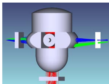
Abb. 6 Der Fluoreszenzdetektor nächster Generation.
