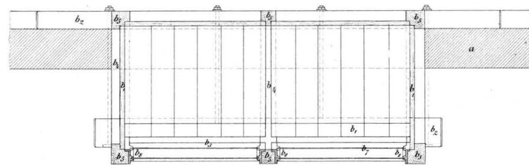
Fig. 4. Horizontal-Durchschnitt des Einlaufes nach i k λ μ
