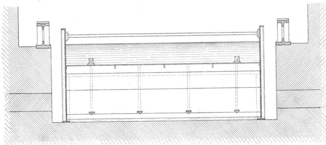
Durchschnitt des Einlaufes
