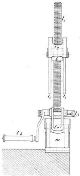
Fig. 3. Ansicht nach der Richtung → Fig. 1
