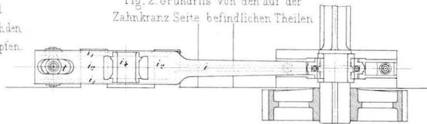
Fig. 9 bis 17 inclusive Hebewerk mit Hängschrauben.
