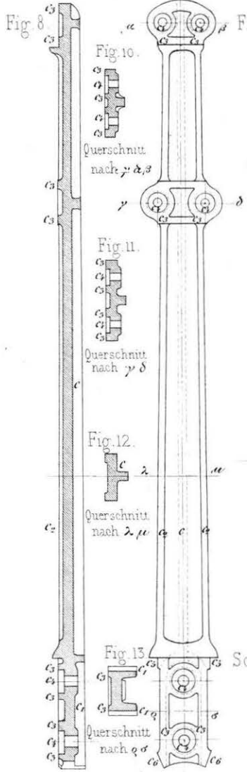
Radarm auf der Zahnkranz Seite Längen Durchschnit
