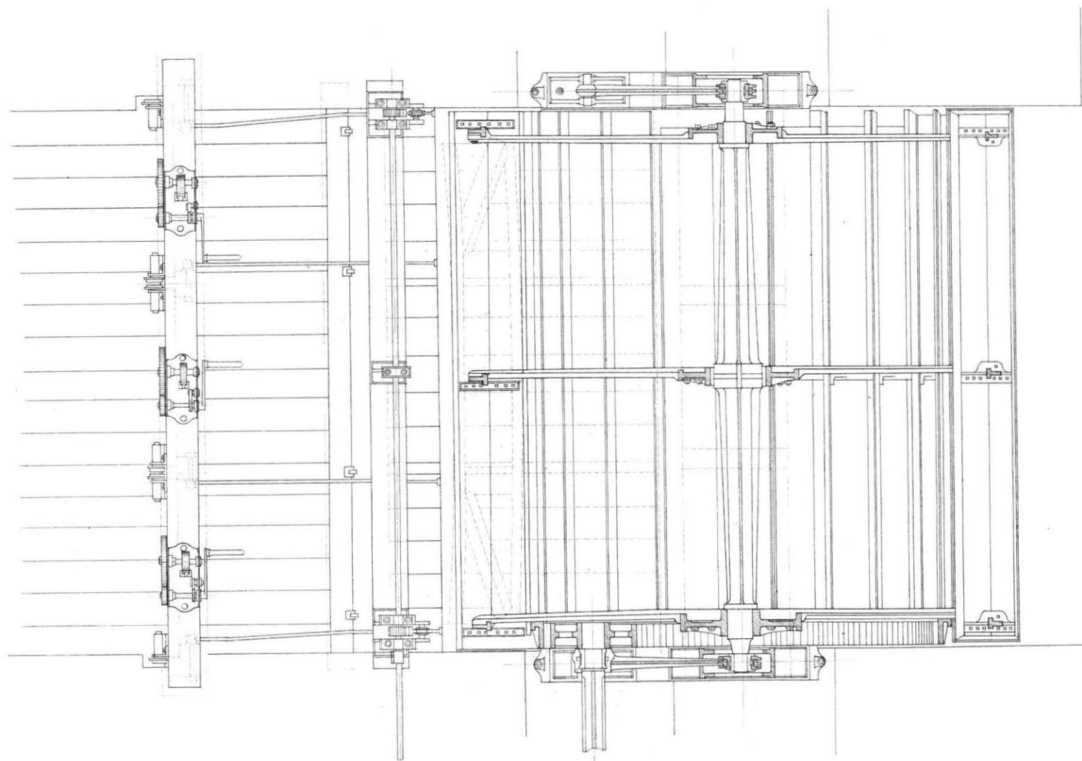
Fig. 2. Grundriß.
