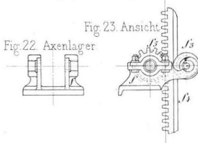
Aufzug für die Regulirschütze
