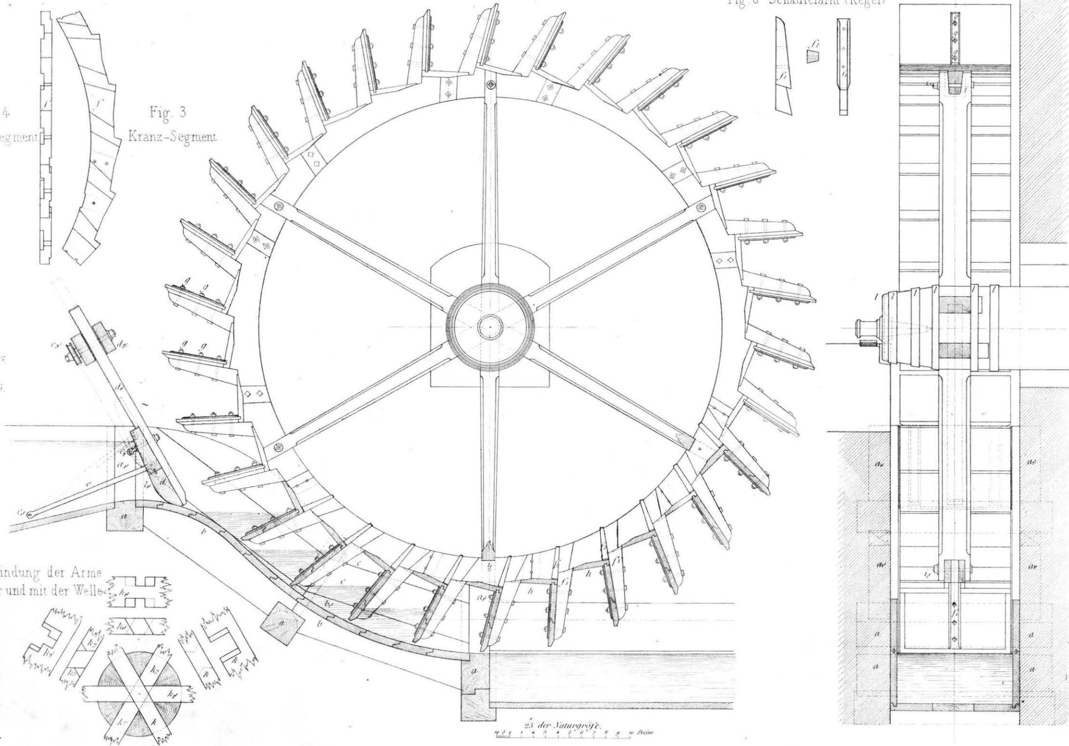
Fig 6 Schaufelarm (Kegel)
