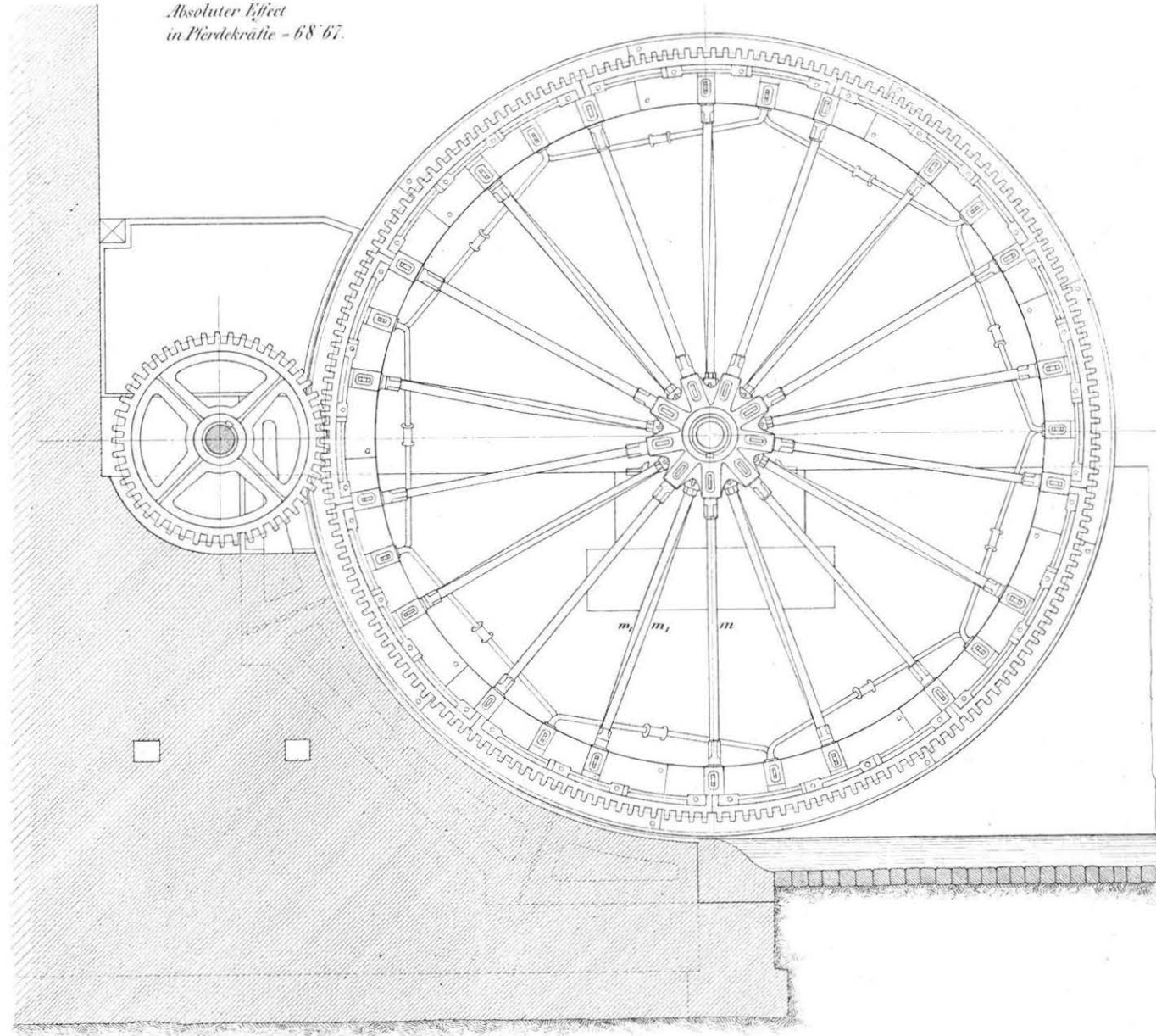
Fig 1 Ansicht des Rades.
