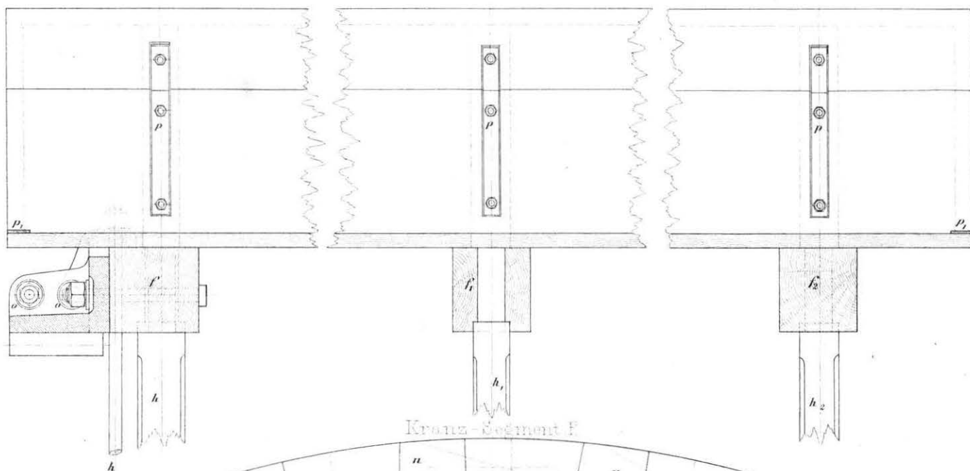
Fig. 2. Verbindung der Kranz Segmente f. concave Seite.
