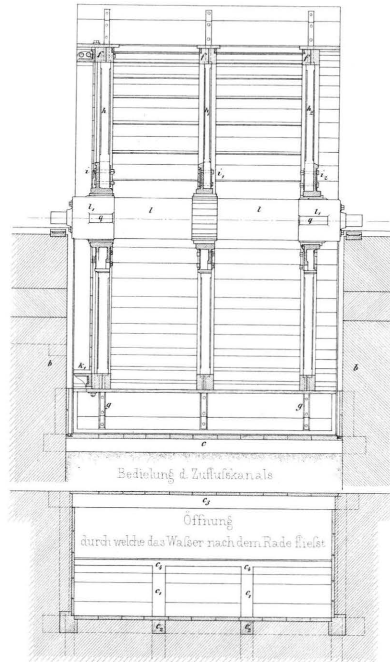
Fig. 4. Vertikalschnitt durch die Kammer vor dem Einlauf nach u.v.w.x. Fig. 1.
