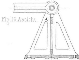
Lagerung des Armes zur Führung der Radwelle auf der dem Zahnkranz gegenüber befindlichen Seite des Rades
