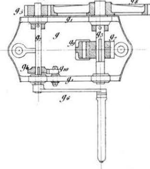
Fig. 22. Grundriß.
