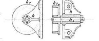
Lauf Rolle zur Einlaß Schleufe.
