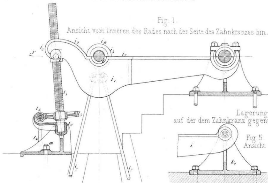
Fig. 1 bis 8 inclusive Hebewerk mit Stützschauben.
