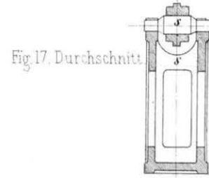
Lagerung des Armes zur Führung der Radwelle auf der dem Zahnkranz gegenüber befindlichen Seite des Rades
