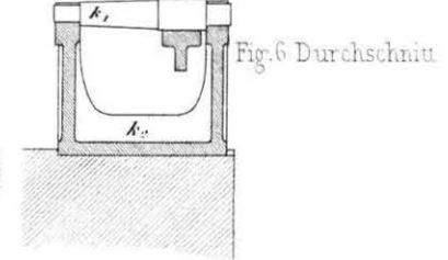
Lagerung des Traghebels auf der dem Zahnkranz gegenüber befindlichen Seite des Rades
