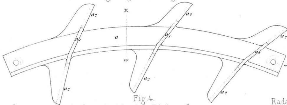
Fig. 4. Außere Ansicht eines Zahnkranz-Segmentes.
