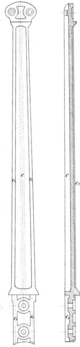
Radarm des mittleren Systemes Fig. 14. Ansicht. Fig. 15. Längen Durchschnit.
