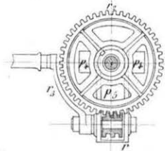
Fig. 12. Grundrifs der Winde.
