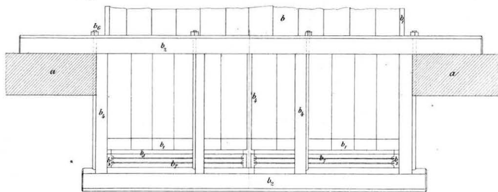
Fig. 3. Horizontal-Ansicht des Einlaufes.
