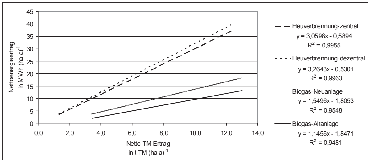
Abbildung 23: Nettoenergieerträge (in MWh ha -1 a -1 ) der Nutzungskonzepte der Energiebereitstellung repräsentativer Dauergrünlandpflanzengesellschaften in Abhängigkeit vom Netto- TM-Ertrag (in t TM ha -1 a -1 )
