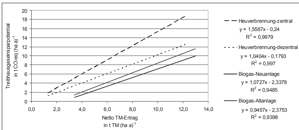
Abbildung 24: Treibhausgaseinsparpotenziale (in t CO 2eq ha -1 a -1 ) der Nutzungskonzepte der Energiebereitstellung repräsentativer Dauergrünlandpflanzengesellschaften in Abhängigkeit vom Netto- TM-Ertrag (in t TM ha -1 a -1 )
