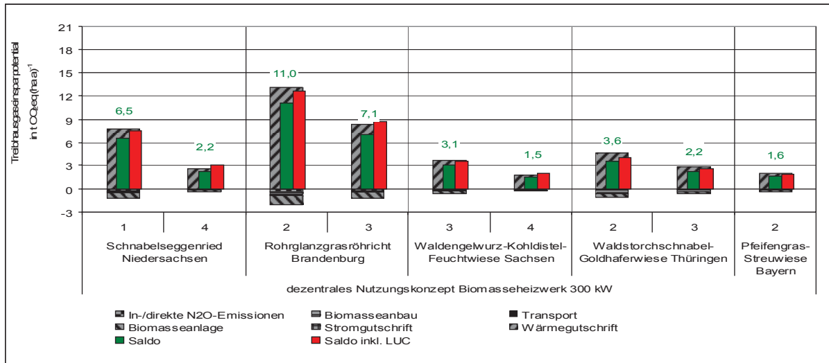
Abbildung 10: Treibhausgasbilanzen und Treibhausgaseinsparpotenziale der Dauergrünlandpflanzengesellschaften im Nutzungskonzept der dezentralen Verbrennung im Biomasseheizwerk 300 kW (LUC = Land Use Change)
