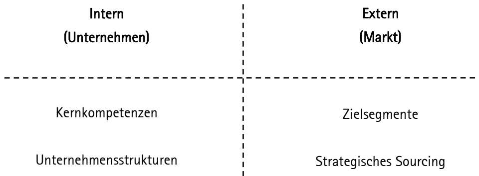
Abbildung 43: Strukturelle Strategiekomponenten
