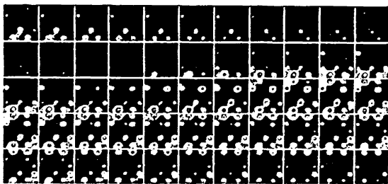
Abb.2: Folge komplexer adaptiver Varianzschätzungen
