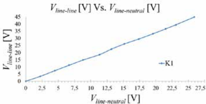
Figura 6. Respuestas del generador con pruebas en vacío
