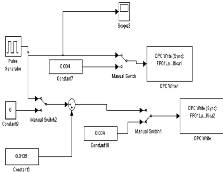
Figura 2. Programa en Simulink
