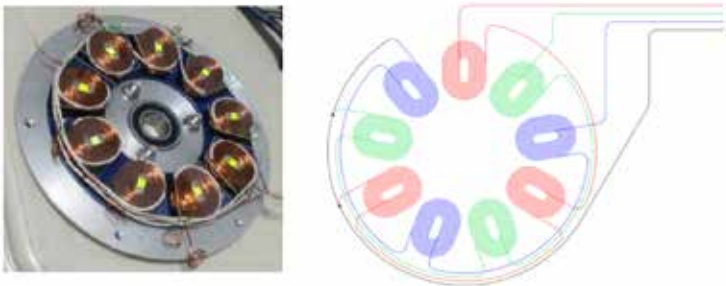
Figura 4. Construcción y conexiones de las bobinas
