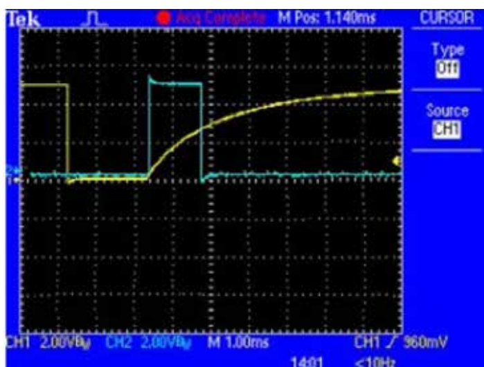
Figura 7. Señales adquiridas del sensor resistivo por medio de un osciloscopio, al levantar 1kg de peso
