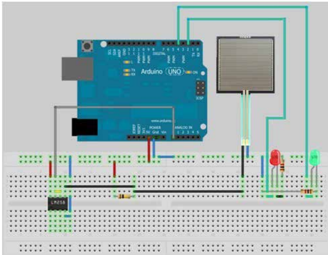
Figura 3. Circuito implementado para el sistema
