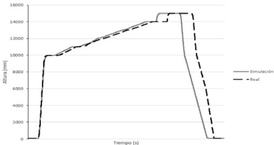
Figura 6. Comparación de estabilidad de la altura
