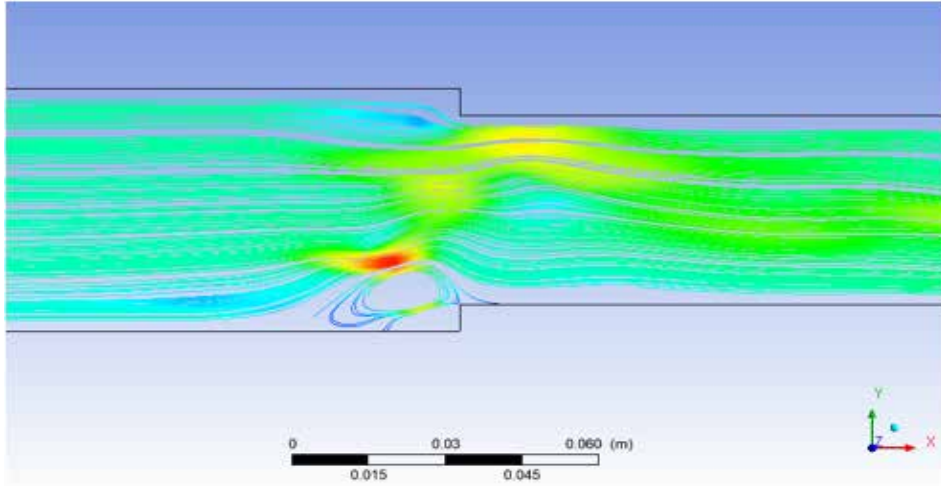
Figura 9. Líneas de flujo de turbulencia
