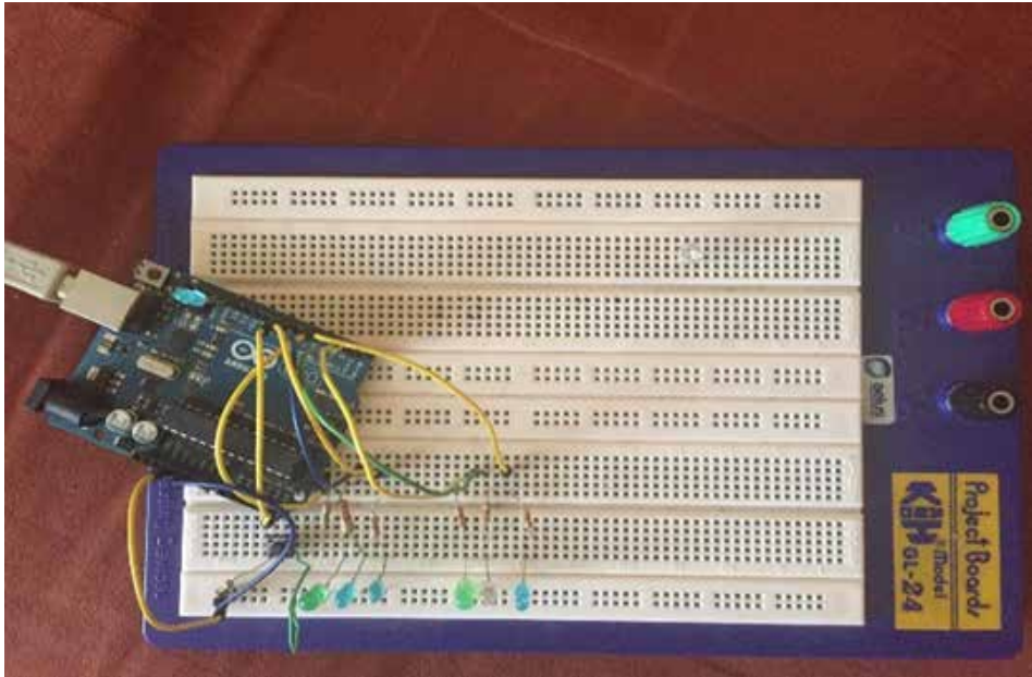
Figura 3. Circuito de comunicación con la tarjeta Arduino
