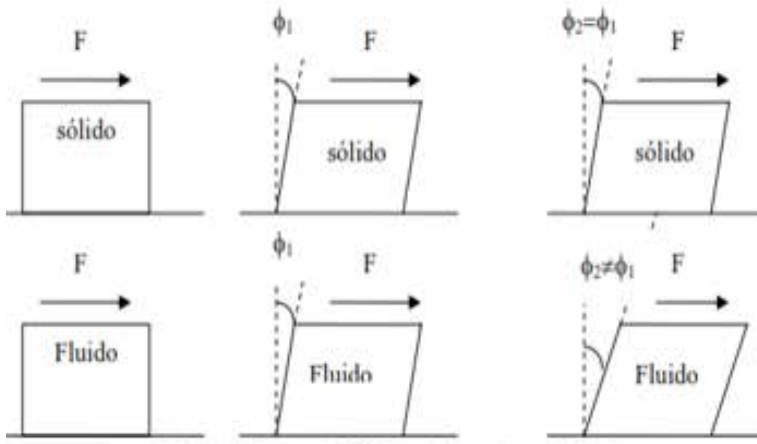
Figura 2. Esfuerzo de Cizallamiento sobre un Sólido y un Fluido
