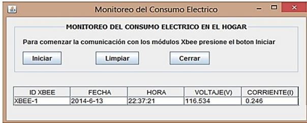
Figura 10. Valor obtenido del voltaje y la corriente consumida de la laptop en el sistema de monitoreo.
