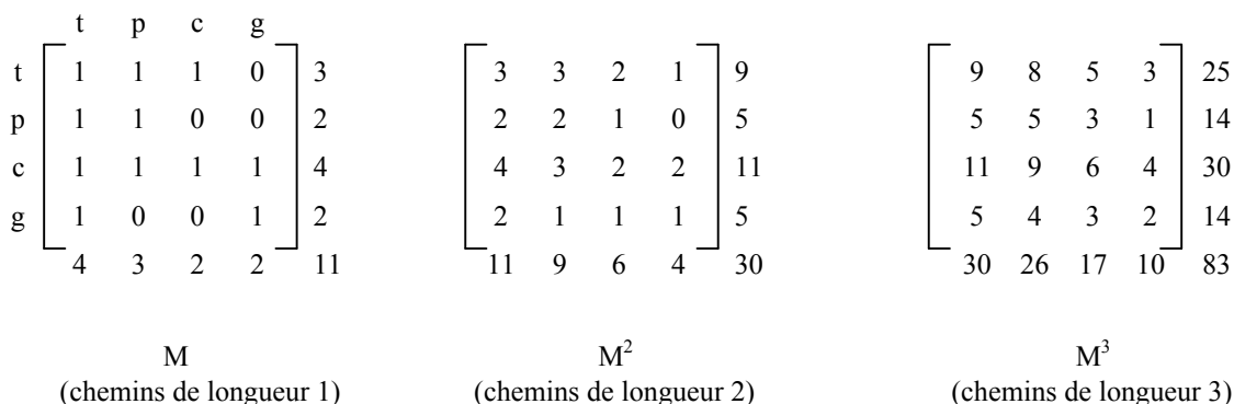
Figure 4. Matrice M associée au graphe G , son carré M^2 et son cube M^3 Il suffit d'arriver à M^3 pour que toutes les liaisons 2 à 2 soient vérifiées : ce réseau facilite grandement les changements de rôles
