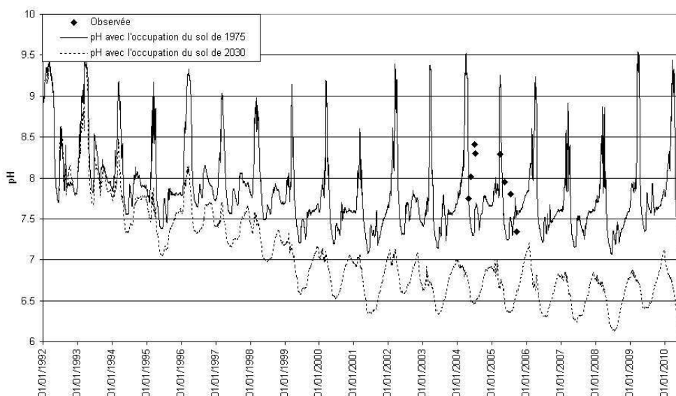
Figure 9 : Évolution du pH des eaux du lac d'Ilay durant la période 1992-2010 avec les modes d'occupation des sols de 1975 et 2030
