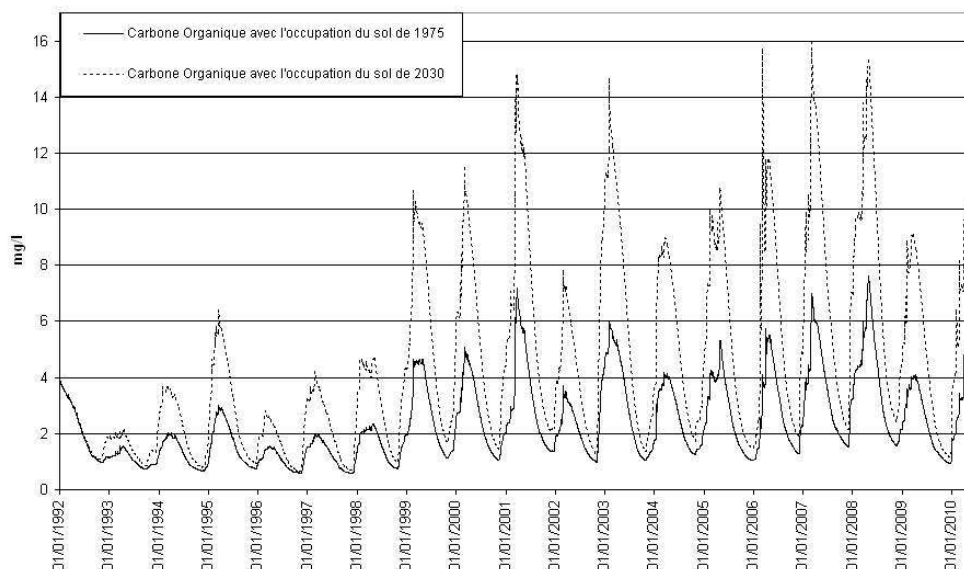
Figure 8 : Comparaison de l'évolution des taux de carbone organique durant la période 1992-2010 avec les modes d'occupation des sols de 1975 et de 2030
