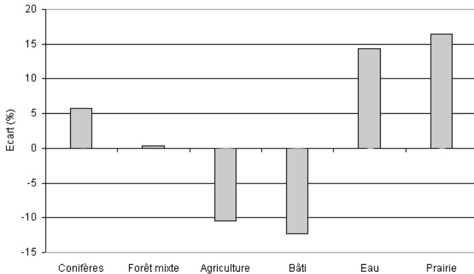
Figure 5 : Écart résiduel (en %) entre les résultats obtenus par télédétection de la photosatellite 2006 et la carte prédictive de 2006
