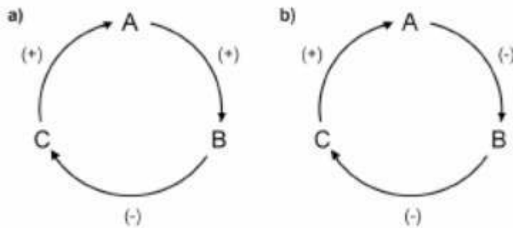
FIGURA 4. ESQUEMA DE CICLOS DE RETROALIMENTACIÓN A) NEGATIVA (“AUTOEQUILIBRANTE”) Y B) POSITIVA (“AUTORREFORZADORA”). EL SIMPLE CAMBIO EN LA POLARIDAD DE UNO DE LOS ENLACES DE CONTROL, CAMBIA LA POLARIDAD DEL CICLO COMPLETO.
