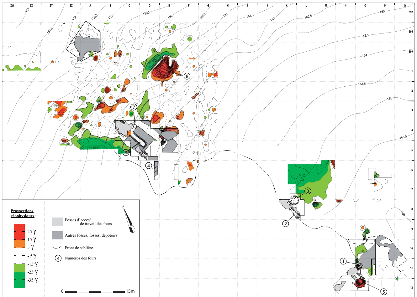
Fig. 16 : Deux exemples d'ateliers ruraux mixtes : ci-dessus : a) plan d'ensemble de l'atelier de Vignny (Loiret), d'après FERDIÈRE, GUILLEMARD et LANOS 2012 : Fig. 3 ; les fours de tuiliers sont ceux du groupe ouest (à gauche), ainsi sans doute que le four 5, en bas à droite (groupe est) ; les autres fours sont de potiers (DAO Th. Guillemard) ; ci-contre, page de droite : b) plan d'ensemble de l'atelier, Les Clouzeaux (Vienne) (DAO F. Sanz Pascual, extr. de SÉRIS 2008).
