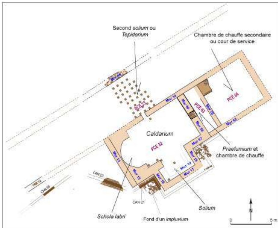
Fig. n°4 : Cheberne : plan de l'ensemble balnéaire annexe
