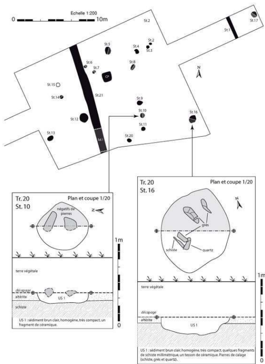
Fig. 2 – Site 1 (site néolithique), structures 10 et 16 : trou de poteau (plan et coupe)
