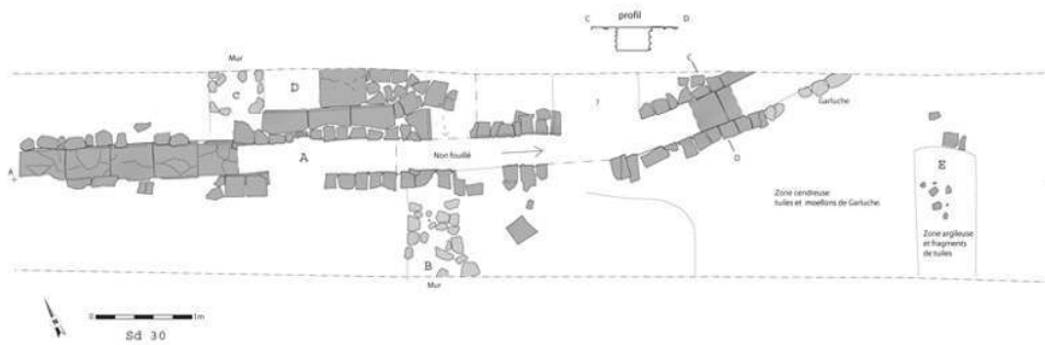
Fig. n°2 : Plan de détail de la structure 30 du sondage 30
