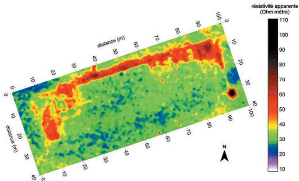
Fig. n°1 : Carte de résistivité apparente d'un secteur de la zone portuaire. Les résistivités élevées indiquent la présence de structures maçonnées
