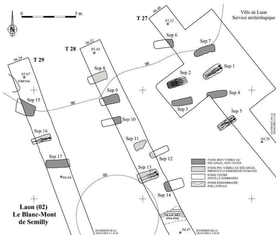
Fig. n°1 : Laon « Le Blanc Mont de Semilly - Résidence Laurence ». Plan des vestiges (J.-P. Jorrand, SA de Laon)
