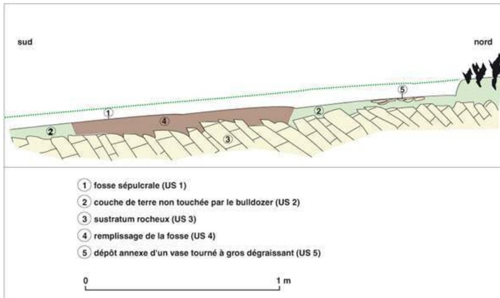
Fig. n°2 : Coupe de la tombe selon l'axe sud-nord
