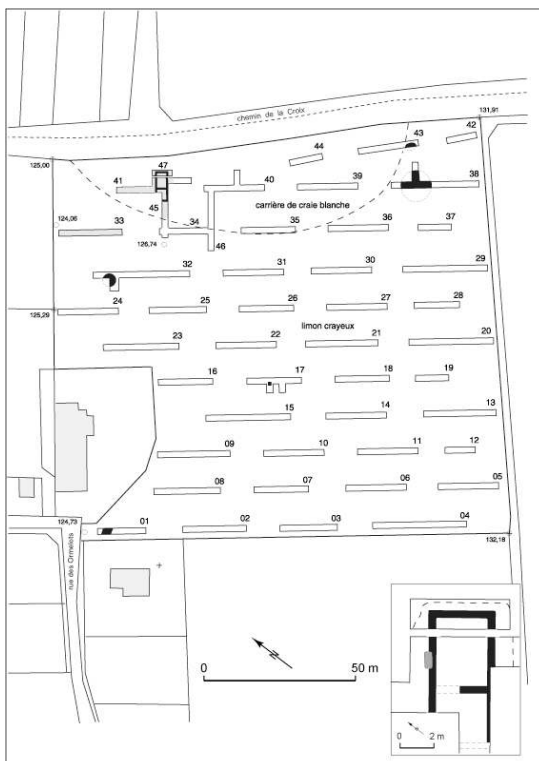
Fig. n°1 : Position des vestiges et plan du bâtiment d'exploitation
